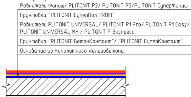
Рис.16. Конструктивный разрез №4.
