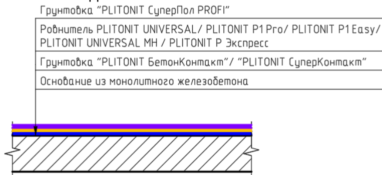
Рис.15. Конструктивный разрез №3.
