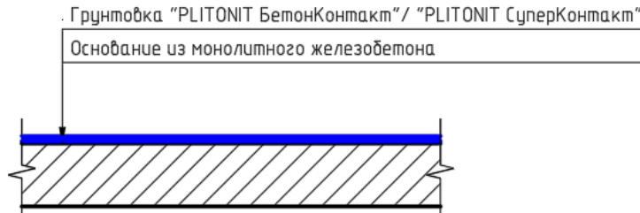
Рис.12. Конструктивный разрез №1.
