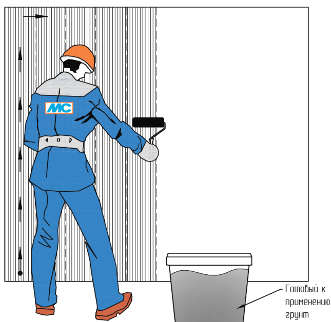
Рис. 6. Схема организации работ по нанесению грунта на основание
