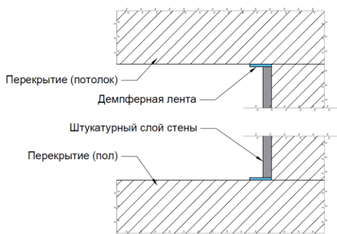
Рис.22. Приклейка демферной ленты в местах сопряжения штукатурного слоя со стеной и потолком
