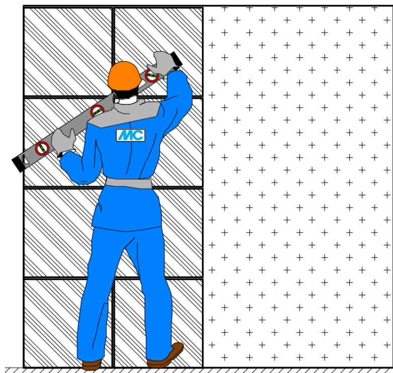
Рис.29. Последовательность работ, где: 1 – проверка ровности основания контрольной рейкой; 2, 3 – приготовление грунтовки; 4 – нанесение грунтовки на цементную штукатурку; 5 – приготовление клеевой смеси; 6, 7 – нанесение клеевой смеси на основание (захватками); 8, 9 – приклеивание керамогранитной плитки на стену (захватками); 10 – проверка облицовки при помощи уровня. ПРИМЕЧАНИЕ к рис 30.: на этапах 6-9 указано проведение работ в направлении снизу вверх, но при использовании клеев, в маркировке которых присутствует буква «Т», возможно выполнение работ в направлении сверху вниз.
