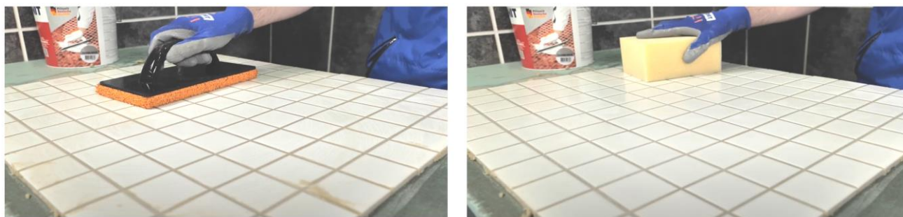
Рис. 34. Диагональными движениями шпателя убрать с поверхности плитки излишки затирки
