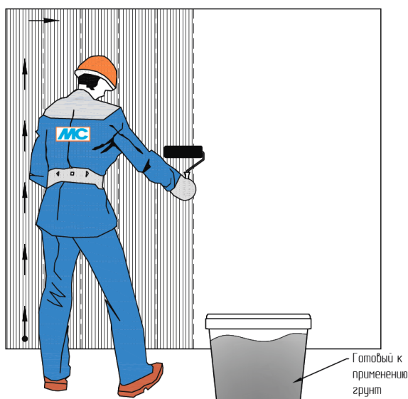
Рис. 21. Схема организации работ по нанесению грунта на основание
