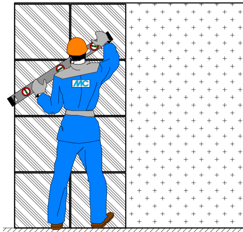
Рис.25. Последовательность работ, где: 1 – проверка ровности основания контрольной рейкой; 2, 3 – приготовление грунтовки; 4 – нанесение грунтовки на цементную штукатурку; 5 – приготовление клеевой смеси; 6, 7 – нанесение клеевой смеси на основание (захватками); 8, 9 – приклеивание керамогранитной плитки на стену (захватками); 10 – проверка облицовки при помощи уровня.
