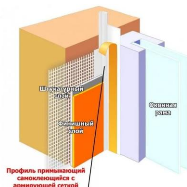
Рис.24. Профиль примыкающий с армирующей сеткой
