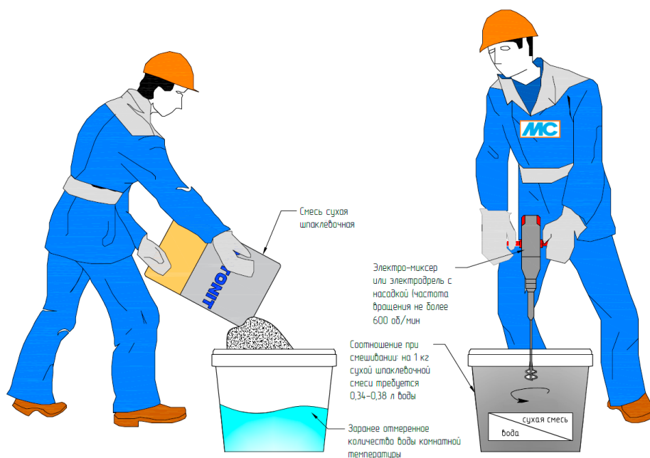
Рис. 30. Организация работ по затворению сухой шпаклевочной смеси
