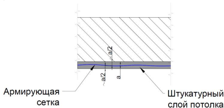
Рис. 13. Армированный штукатурный слой в местах стыка разных материалов и плит перекрытия
