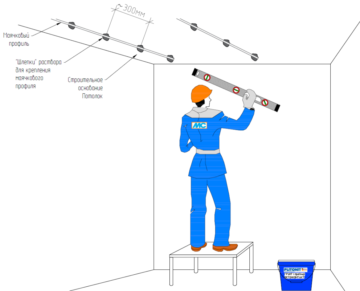
Рис.11. Монтаж маяка с помощью правила с уровнем
