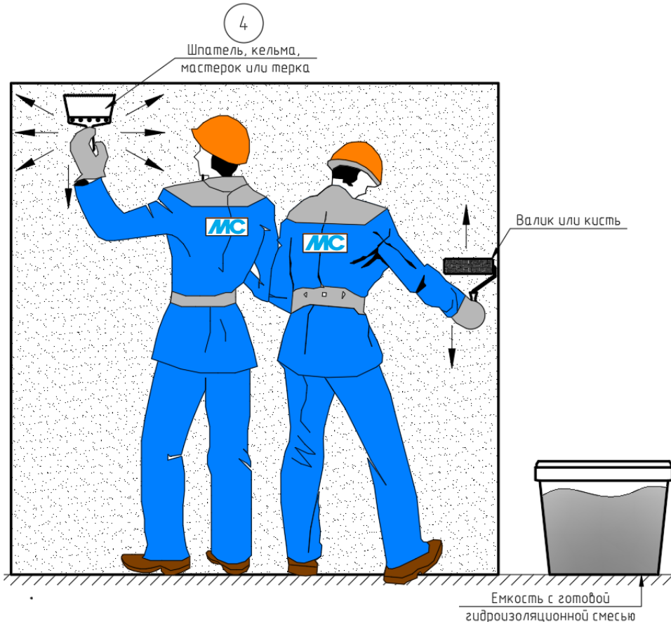
Рис.1. Последовательность работ, где: 1 - проверка ровности основания контрольной рейкой (аналогично для горизонтальной поверхности); 2 – размешивание емкости с мастикой после размораживания до однородной консистенции с использованием дрели с насадкой. В случае, если замораживания не было, предварительное перемешивание мастики не требуется; 3 и 4 – нанесение мастики в 2-3 слоя на основание.
