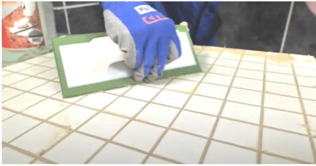
Рис. 38. Диагональными движениями шпателя убрать с поверхности плитки излишки затирки
