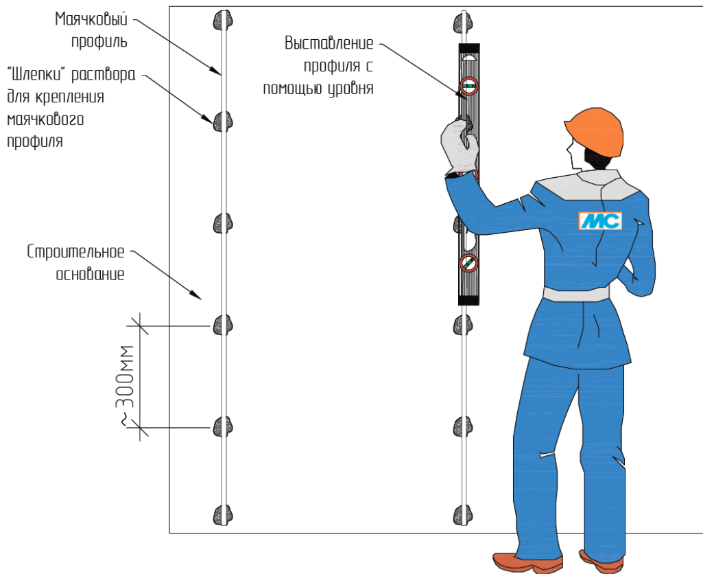
Рис.21. Монтаж маяка с помощью правила с уровнем
