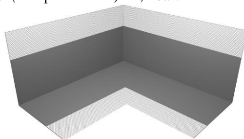
Рис.13. Гидроизоляционный угол «PLITONIT ГидроЛента угол внутренний 90°».
