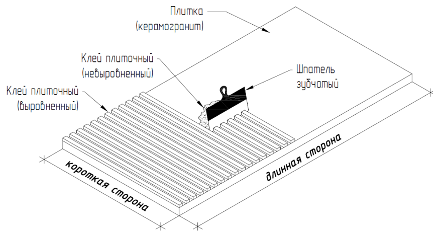
Рис. 34. Нанесение плиточного клея на плитку
