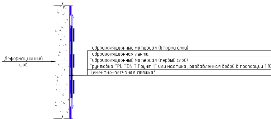
Рис.32.3. Конструктивный разрез №3.
