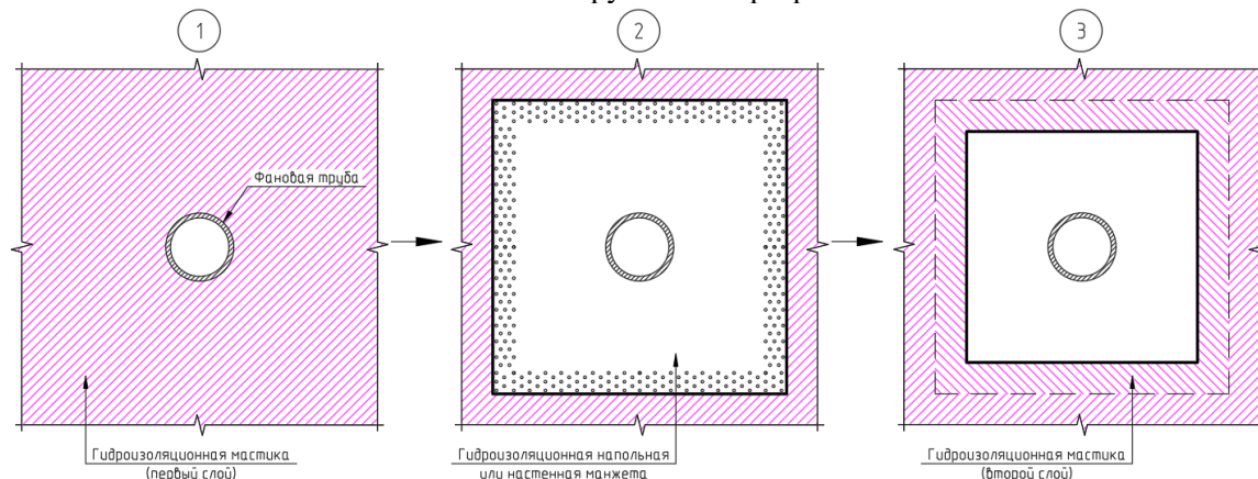
Рис.32.4. Последовательность нанесения гидроизоляционной манжеты.
