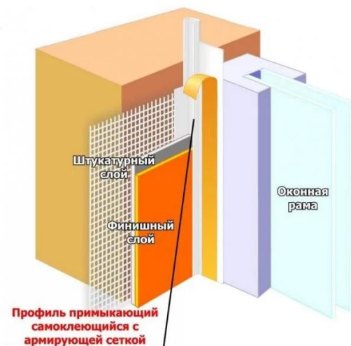
Рис.26. Профиль примыкающий с армирующей сеткой
