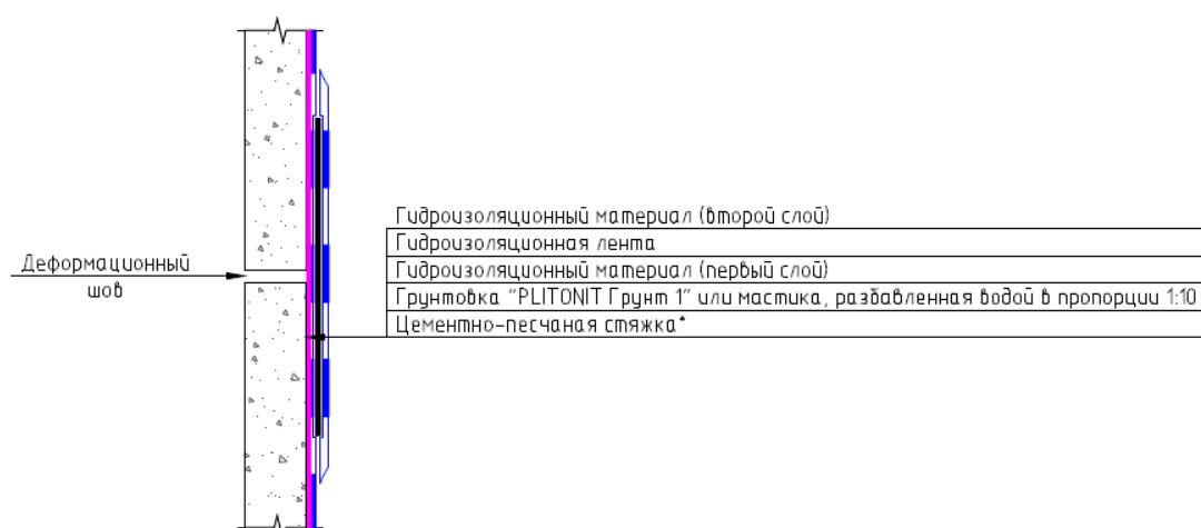
Рис.35.3. Конструктивный разрез №3.
