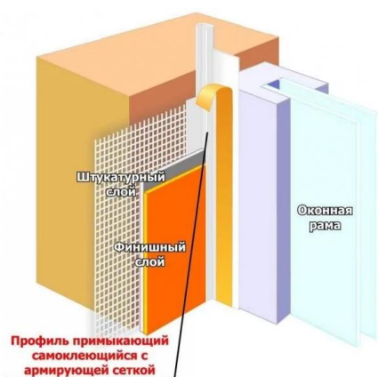
Рис.29. Профиль примыкающий с армирующей сеткой
