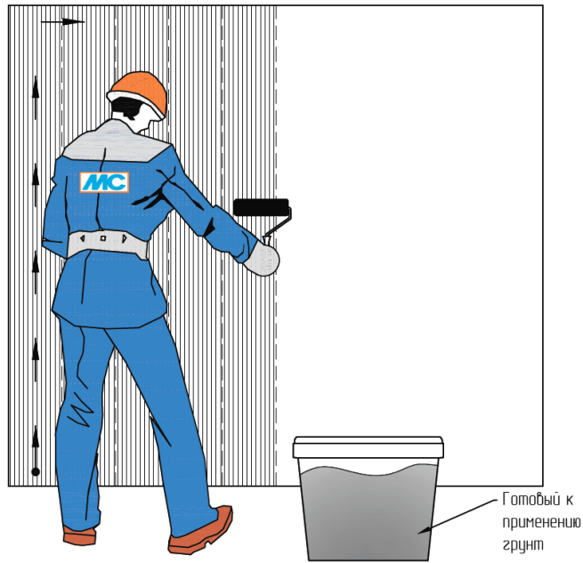
Рис. 33. Схема организации работ по нанесению грунта на основание
