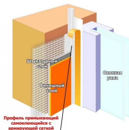
Рис.28. Профиль примыкающий с армирующей сеткой
