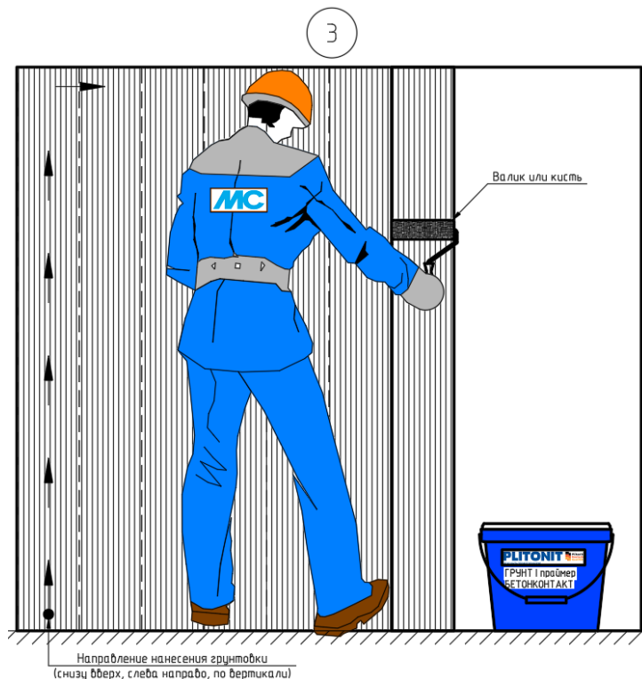
Рис.23. Последовательность работ
