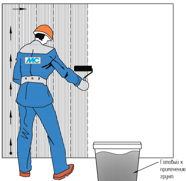
Рис. 6. Схема организации работ по нанесению грунта на основание
