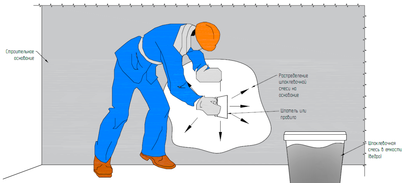
Рис. 8. Организация работ по нанесению шпаклевочной смеси
