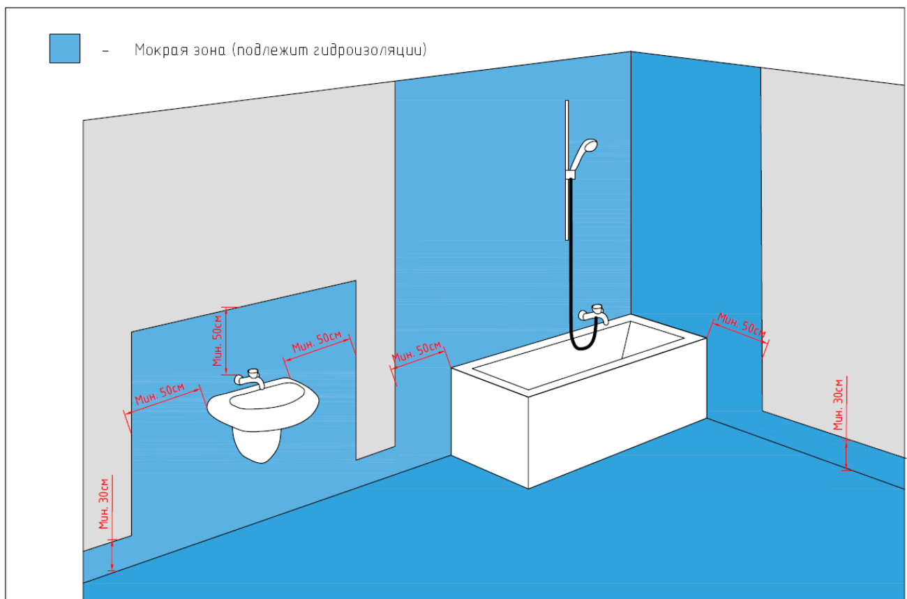
Рис. 14.2 Мокрые зоны внутри влажных помещений, подлежащие гидроизоляции.
