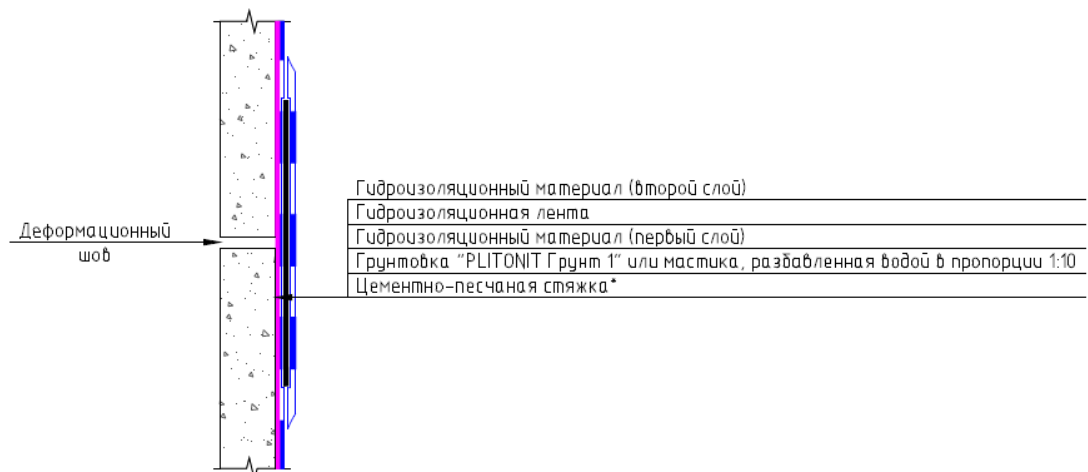
Рис.13.3. Конструктивный разрез №3.
