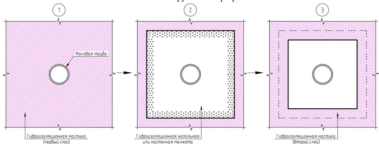
Рис.13.4. Последовательность нанесения гидроизоляционной манжеты.
