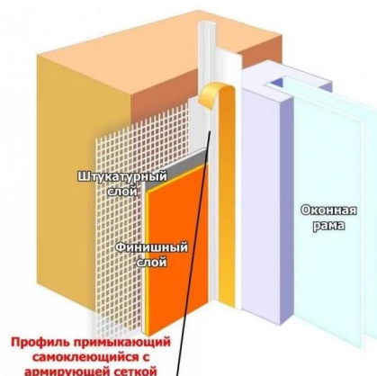
Рис.25. Профиль примыкающий с армирующей сеткой
