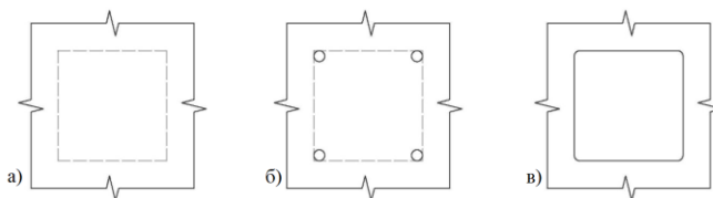
Рис. 36. Резка прямоугольных отверстий
