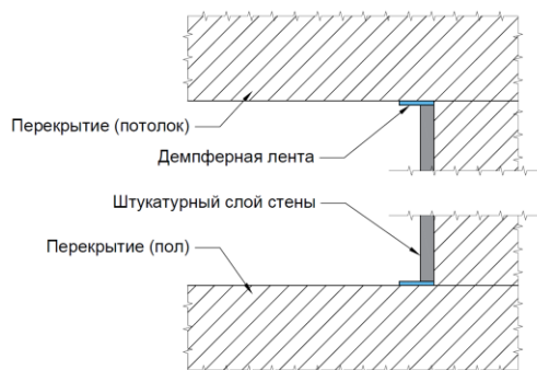
Рис.12. Приклейка демпферной ленты в местах сопряжения штукатурного слоя со стеной и потолком
