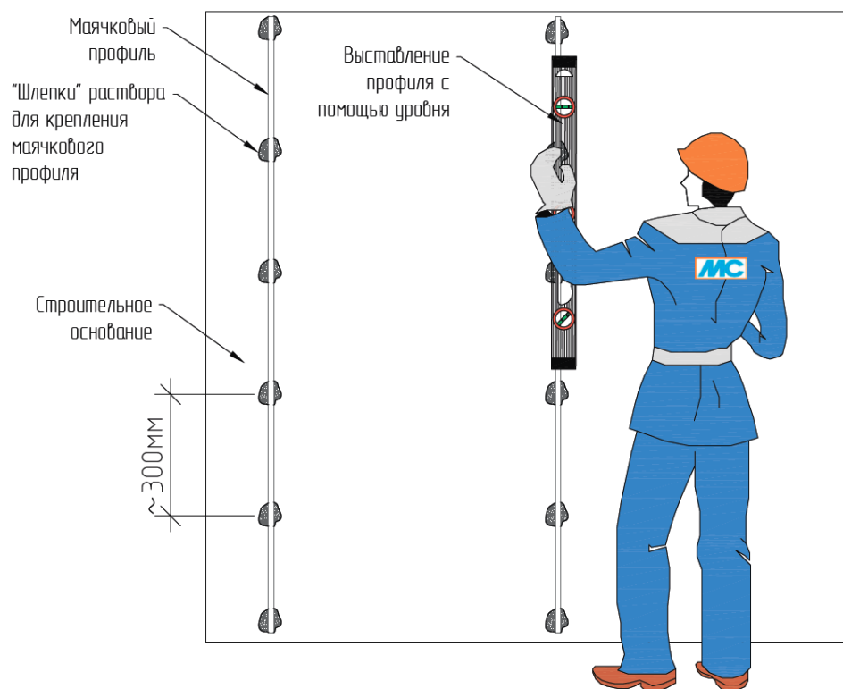
Рис.10. Монтаж маяка с помощью правила с уровнем
