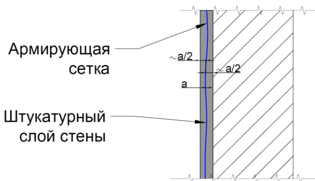
Рис. 16. Армированный штукатурный слой в местах стыка разных материалов стен
