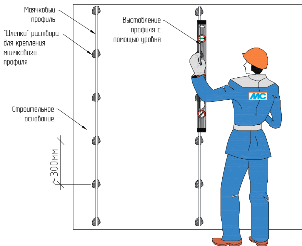
Рис.22. Монтаж маяка с помощью правила с уровнем
