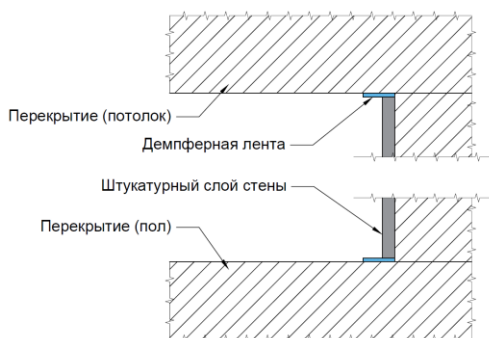
Рис.27. Приклейка демпферной ленты в местах сопряжения штукатурного слоя со стеной и потолком
