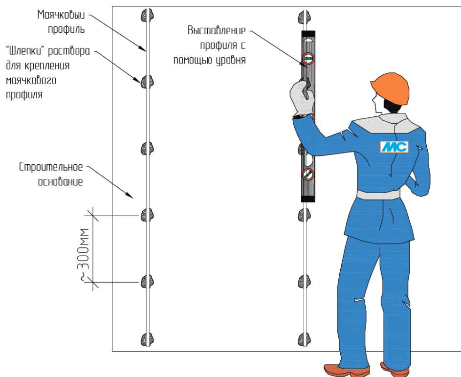
Рис.25. Монтаж маяка с помощью правила с уровнем
