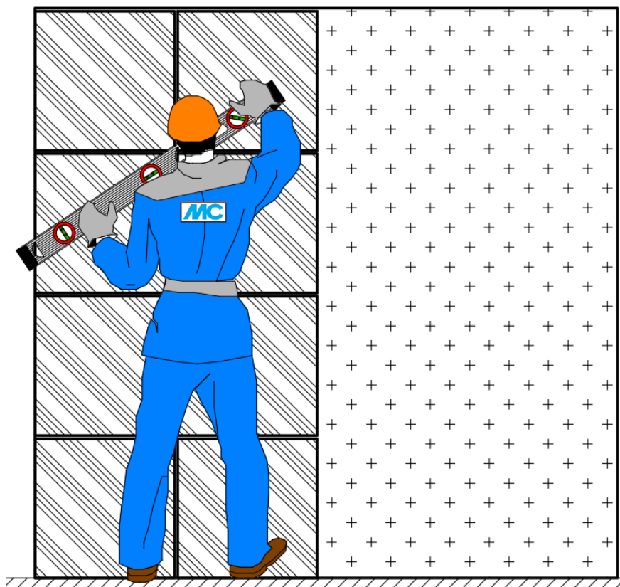
Рис.36. Последовательность работ, где: 1 – проверка ровности основания контрольной рейкой; 2, 3 – приготовление грунтовки; 4 – нанесение грунтовки на цементную штукатурку; 5 – приготовление клеевой смеси; 6, 7 – нанесение клеевой смеси на основание (захватками); 8, 9 – приклеивание керамогранитной плитки на стену (захватками); 10 – проверка облицовки при помощи уровня. ПРИМЕЧАНИЕ к рис 35.: на этапах 6-9 указано проведение работ в направлении снизу вверх, но при использовании клеев, в маркировке которых присутствует буква «Т», возможно выполнение работ в направлении сверху вниз.
