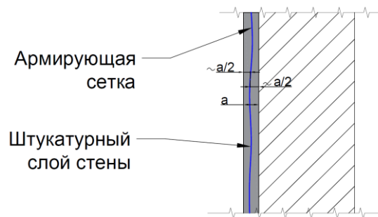
Рис. 31. Армированный штукатурный слой в местах стыка разных материалов стен
