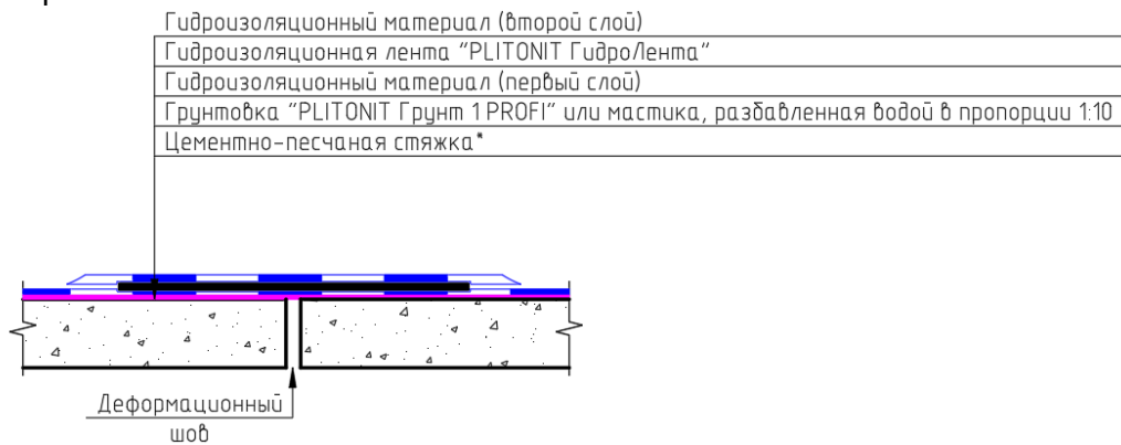
Рис.30. Конструктивный разрез №6.
