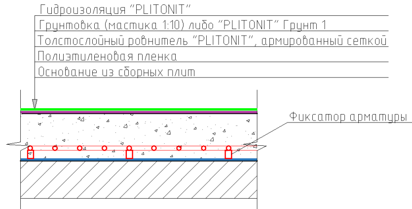
Рис.26. Конструктивный разрез №3
