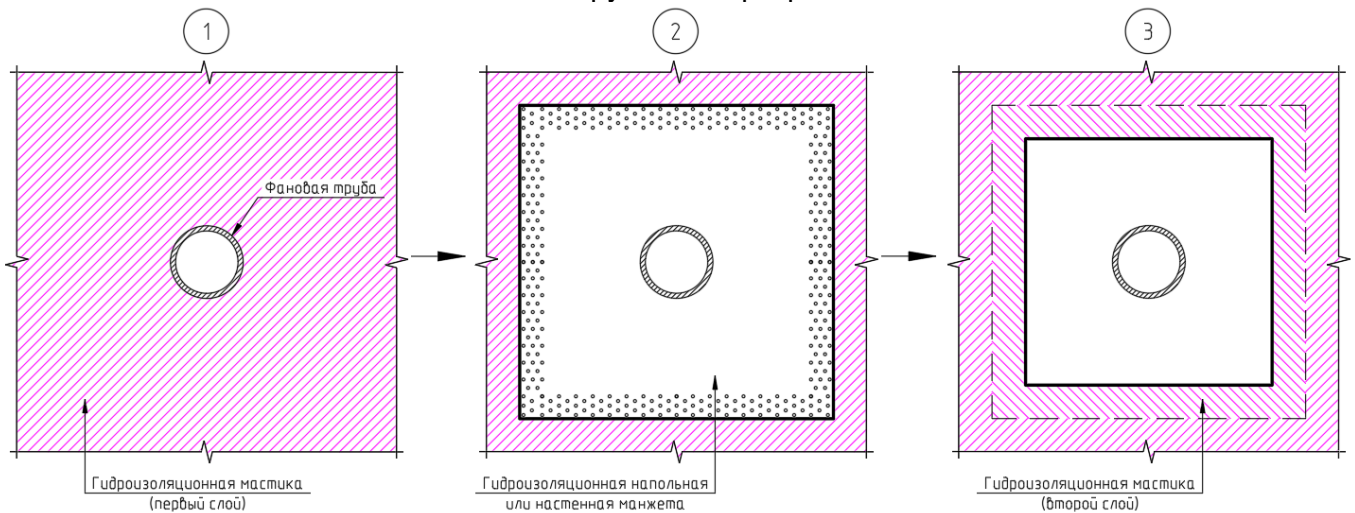
Рис.31. Последовательность нанесения гидроизоляционной манжеты.
