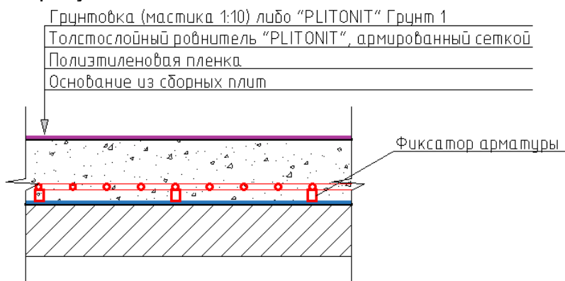
Рис.25. Конструктивный разрез №2.
