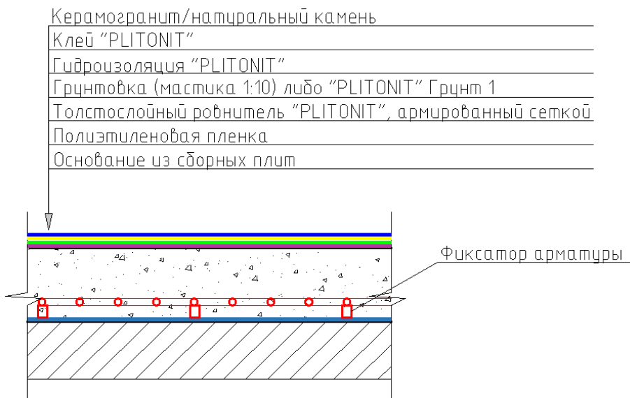
Рис.32. Конструктивный разрез №7.
