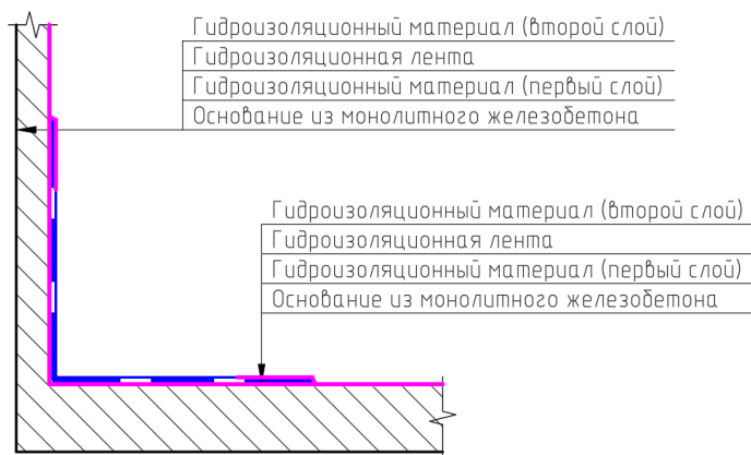
Рис.27. Устройство гидроизоляции внутренних углов с применением «PLITONIT ГидроЛента» и «PLITONIT ГидроЛента угол внутренний 90°».
