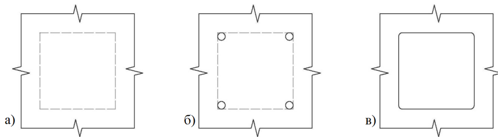
Рис. 36. Резка прямоугольных отверстий
