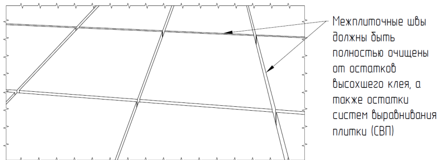
Рис. 40. Подготовка межплиточных швов
