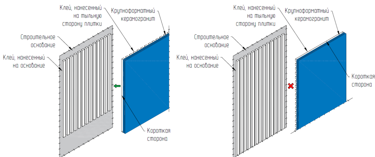
Рис. 33. Клей следует наносить в одном направлении на основание и на плитку
