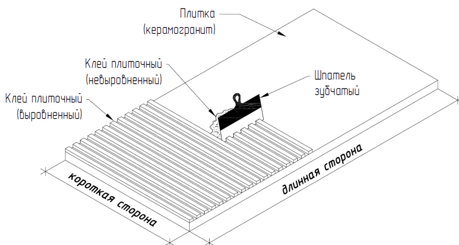
Рис. 32. Нанесение плиточного клея на плитку
