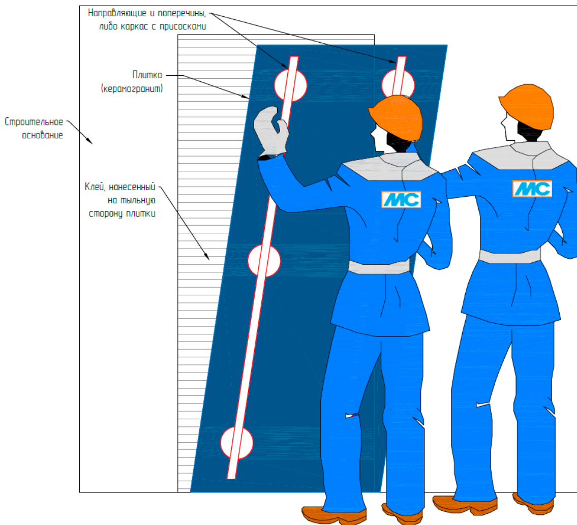
Рис. 37. Монтаж крупноформатного керамогранита
