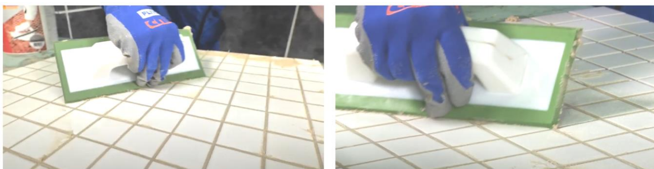
Рис. 43. Диагональными движениями шпателя убрать с поверхности плитки излишки затирки
