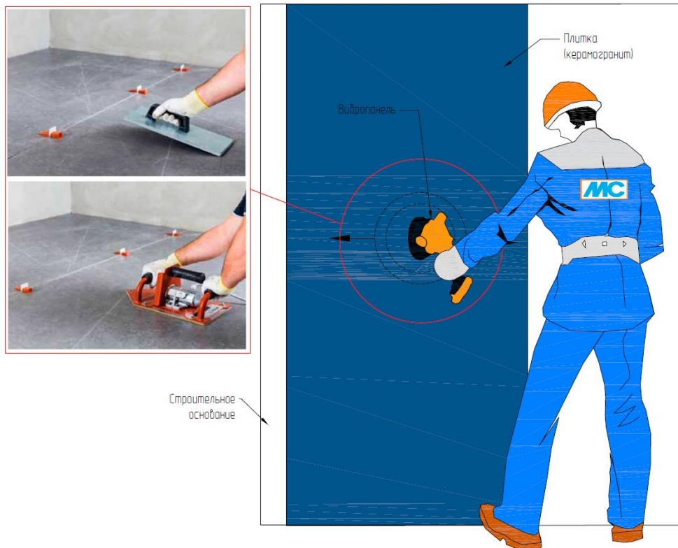
Рис. 38. Увеличение адгезии плитки с основанием вибрированием или простукиванием
