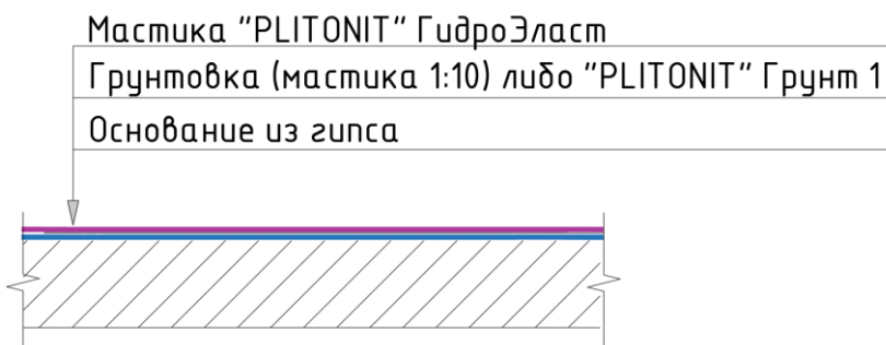
Сечение готового покрытия гидроизоляции.
