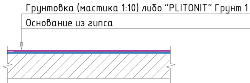
Сечение готового огрунтованного покрытия.
