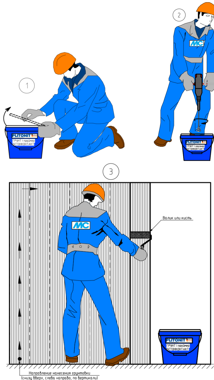
Рис.23. Последовательность работ
