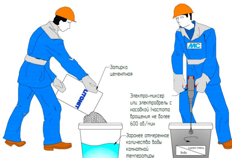
Рис. 37. Приготовление состава
