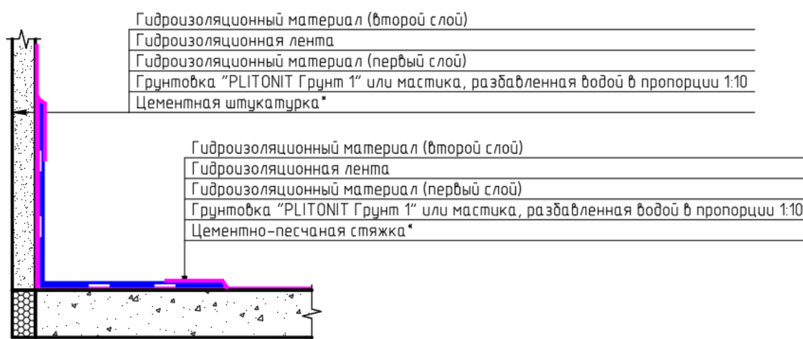
Разрез 1-1
