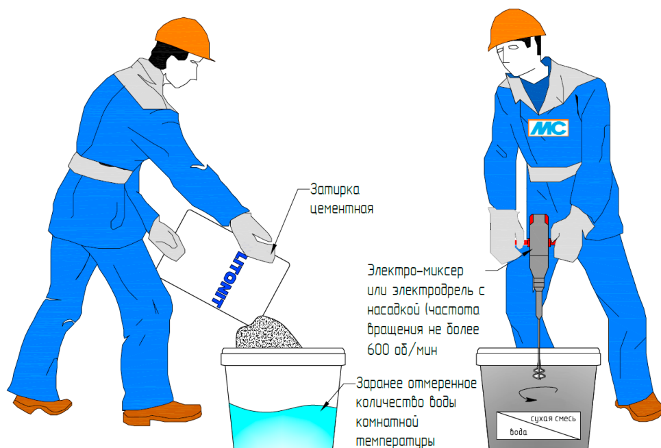
Рис. 29. Приготовление состава
