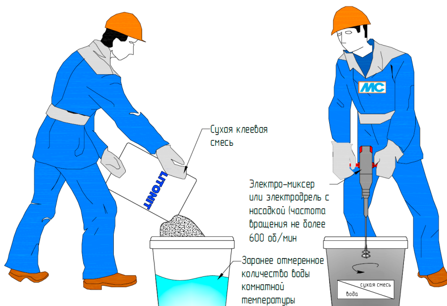
Рис. 26. Организация работ по затворению сухой клеевой смеси
