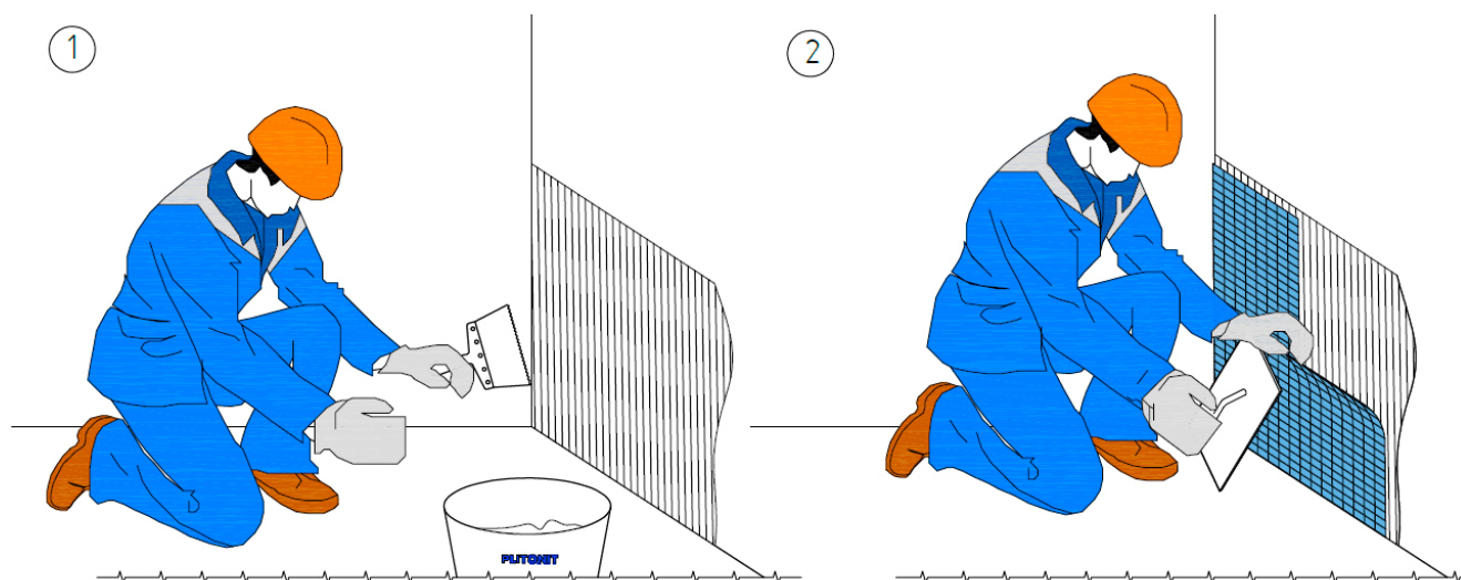
Рис. 27. Организация работ по приклеиванию мозаики
