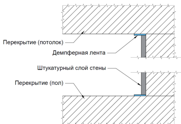
Рис.18. Приклейка демпферной ленты в местах сопряжения штукатурного слоя со стеной и потолком
