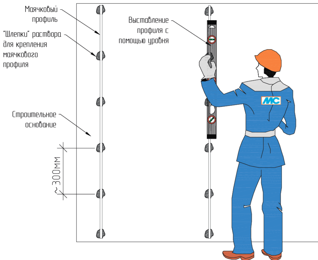
Рис.16. Монтаж маяка с помощью правила с уровнем
