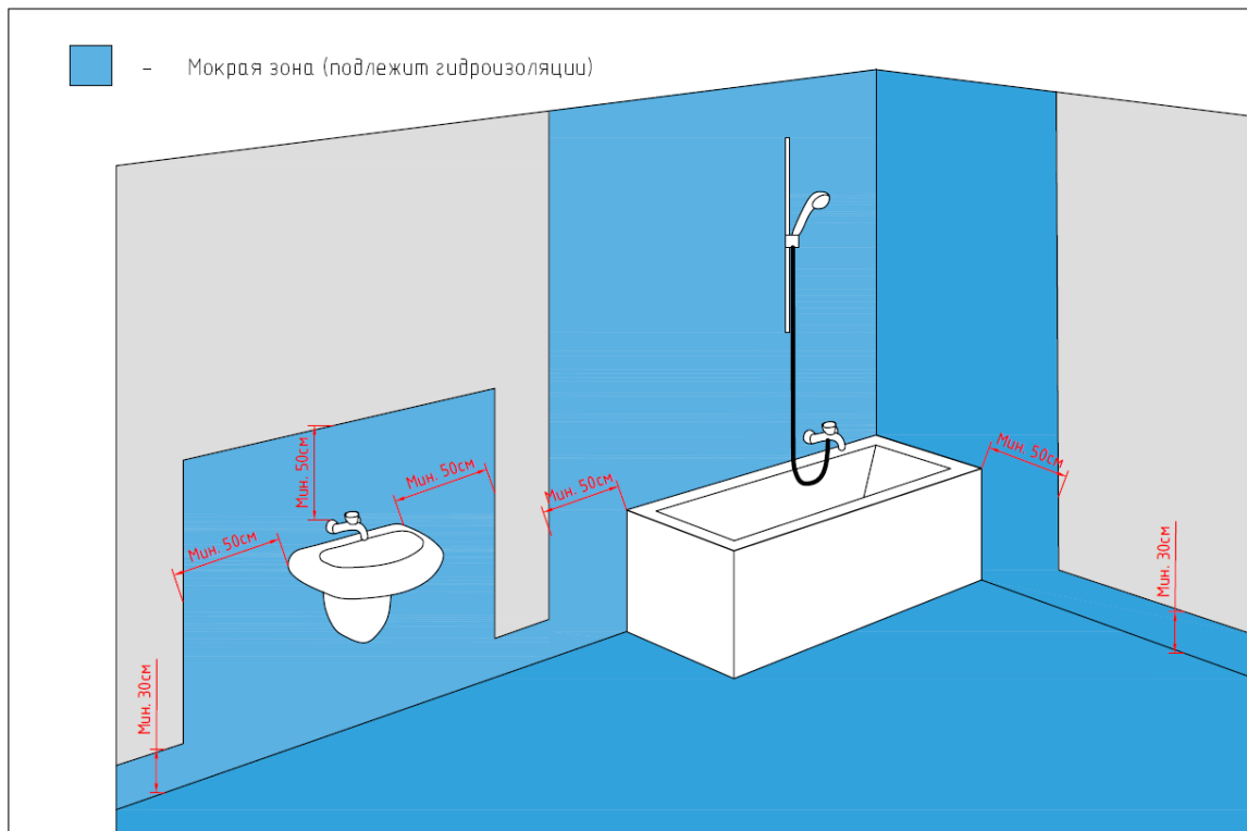
Рис. 23.2 Мокрая зоны внутри влажных помещений, подлежащие гидроизоляции.
