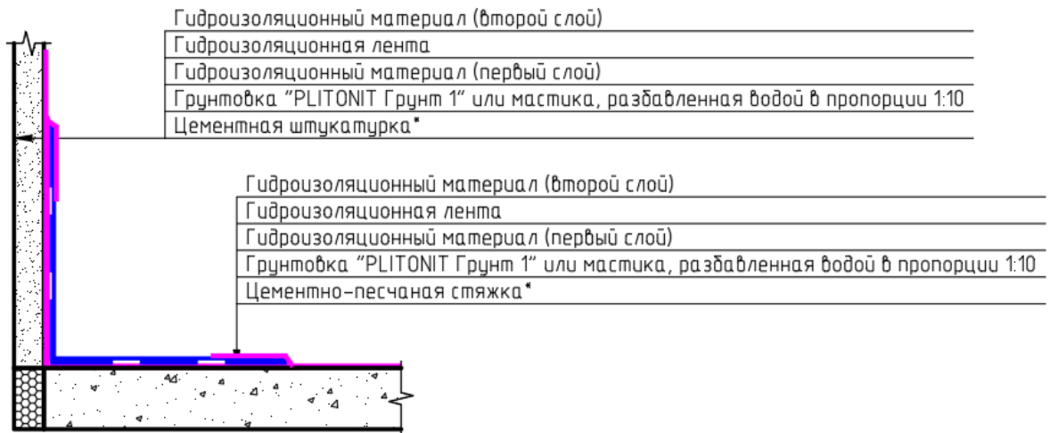
Разрез 1-1
