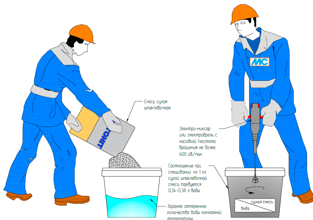
Рис. 15. Организация работ по затворению сухой шпаклевочной смеси
