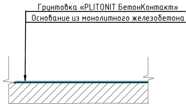
Сечение пирога пола.
