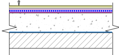
Сечение готового покрытия.
