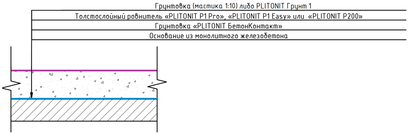
Сечение готового огрунтованного покрытия.
