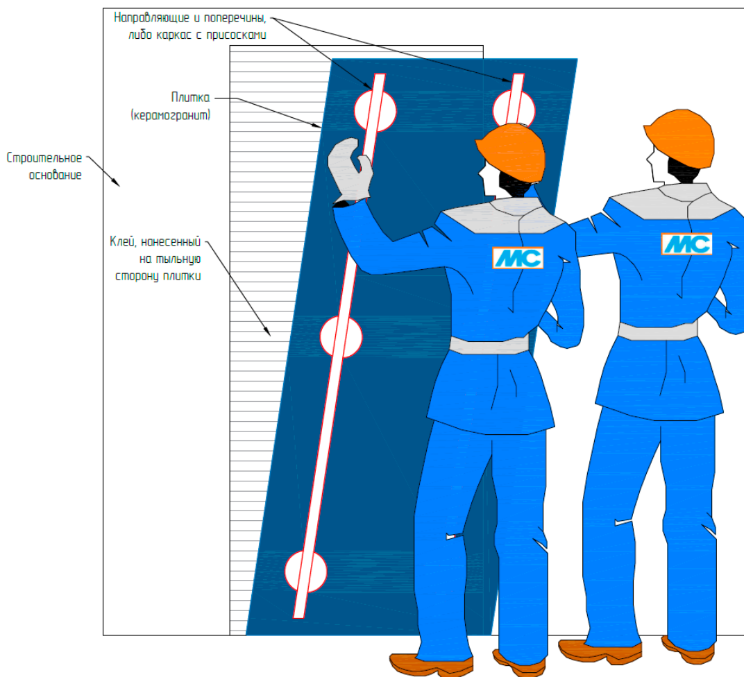
Рис. 18. Монтаж крупноформатного керамогранита
