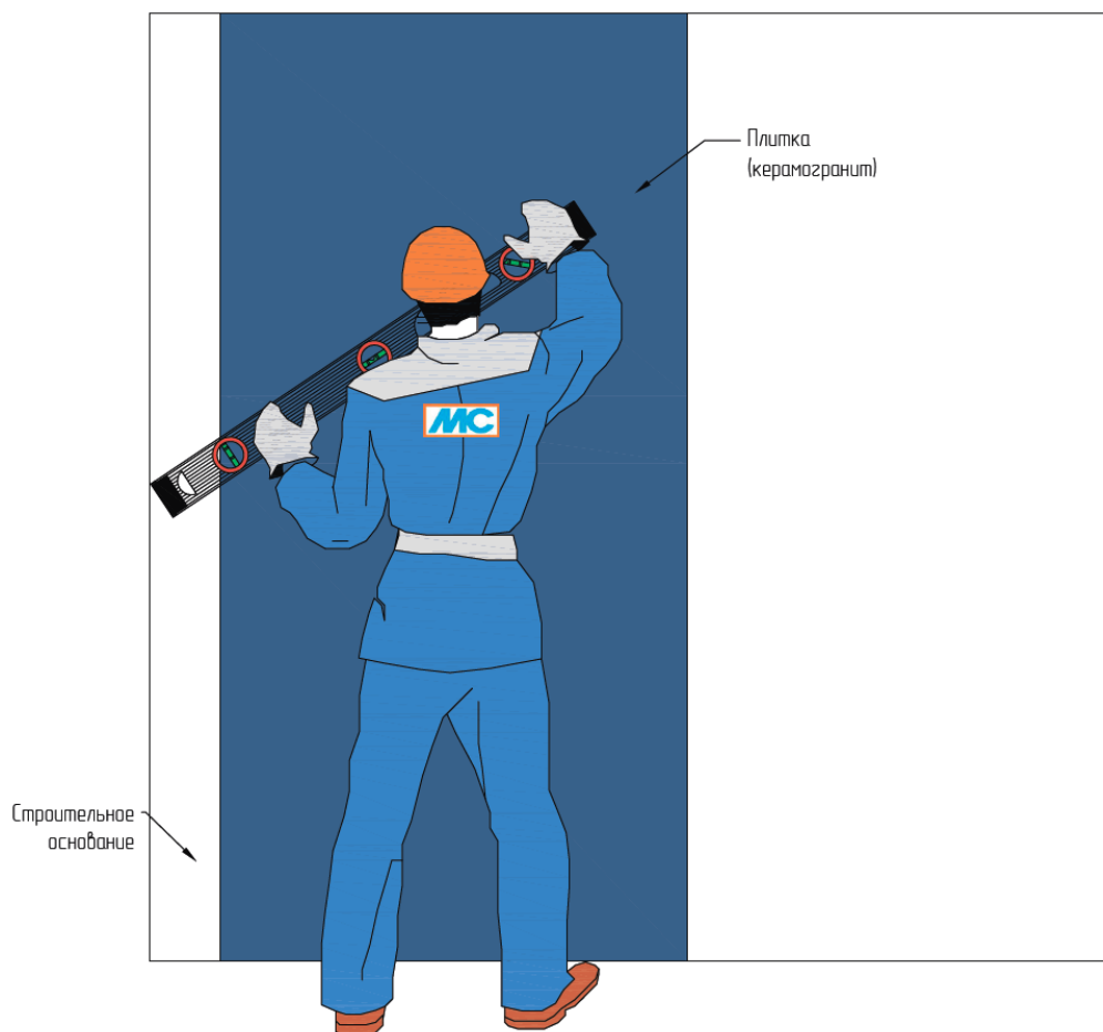
Рис. 20. Проверка облицовки при помощи уровня
