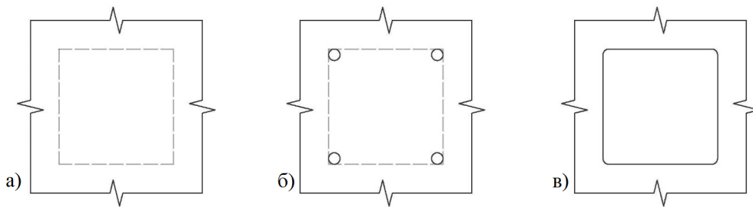
Рис. 17. Резка прямоугольных отверстий
