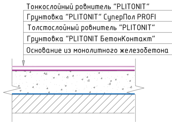
Сечение готового покрытия тонкослойного ровнителя.
