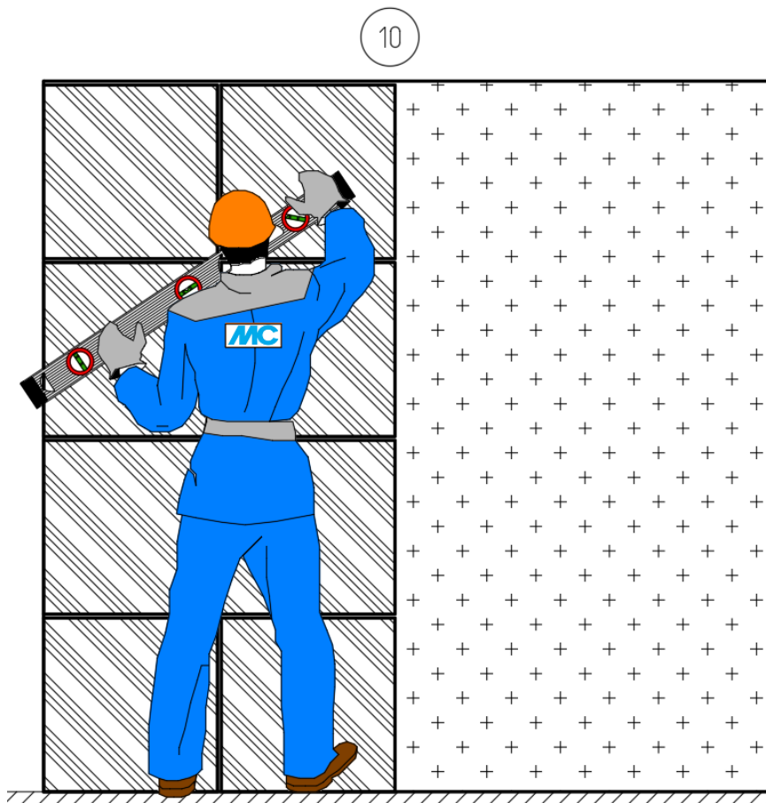
Рис.36.3. Последовательность работ, где: 1 – проверка ровности основания контрольной рейкой; 2, 3 – приготовление грунтовки; 4 – нанесение грунтовки на цементную штукатурку; 5 – приготовление клеевой смеси; 6, 7 – нанесение клеевой смеси на основание (захватками); 8, 9 – приклеивание керамогранитной плитки на стену (захватками); 10 – проверка облицовки при помощи уровня.
