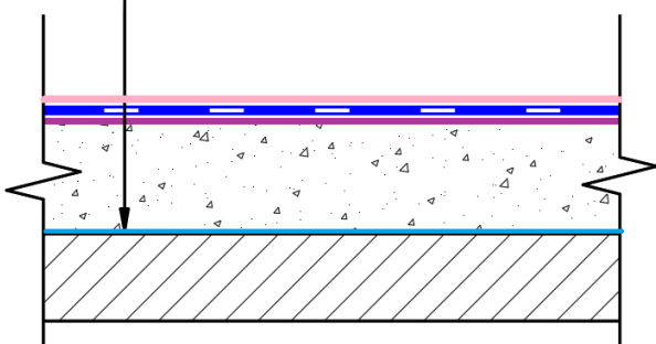
Сечение готового покрытия тонкослойного ровнителя.
