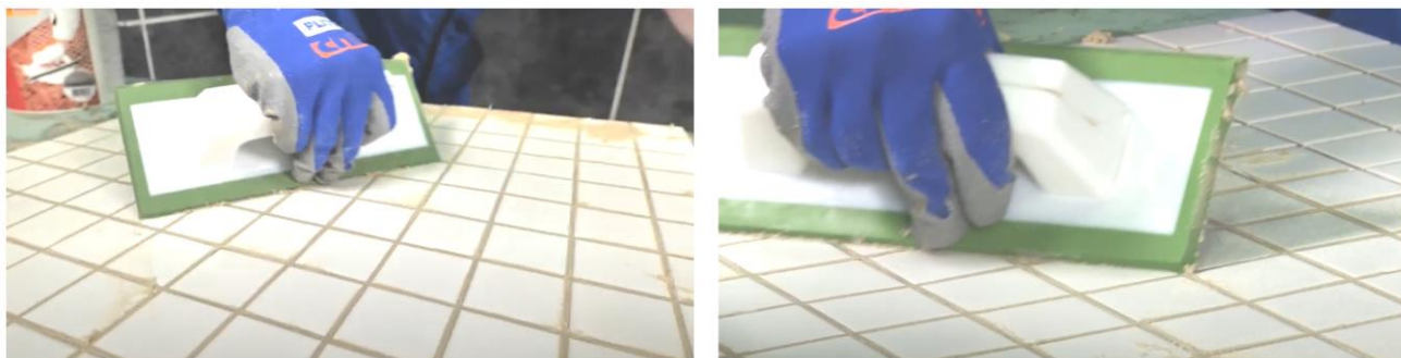
Рис. 26. Диагональными движениями шпателя убрать с поверхности плитки излишки затирки
