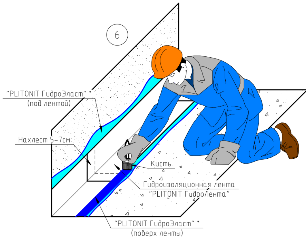
Рис.18. Последовательность работ, где: 1 - проверка ровности основания контрольной рейкой (аналогично для горизонтальной поверхности); 2 – размешивание емкости с мастикой; 3 – нанесение первого слоя мастики, разбавленной водой в пропорции 1:10, на основание; 4 – нанесение гидроизоляции на поверхность (аналогично для горизонтальной поверхности); 5 – укладка гидроизоляционной ленты на поверхность, предварительно обработанную «PLITONIT ГидроЭласт» или «PLITONIT WaterProof Standard»; 6 – поверхностная обработка ленты мастикой «PLITONIT ГидроЭласт» или «PLITONIT WaterProof Standard».
