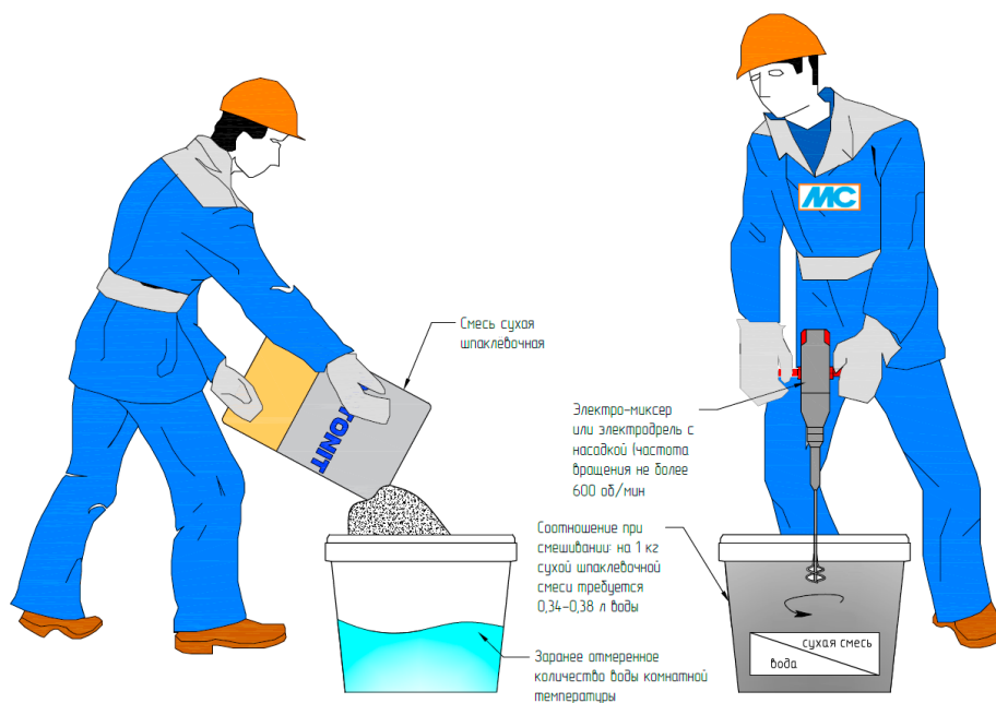
Рис. 19. Организация работ по затворению сухой шпаклевочной смеси
