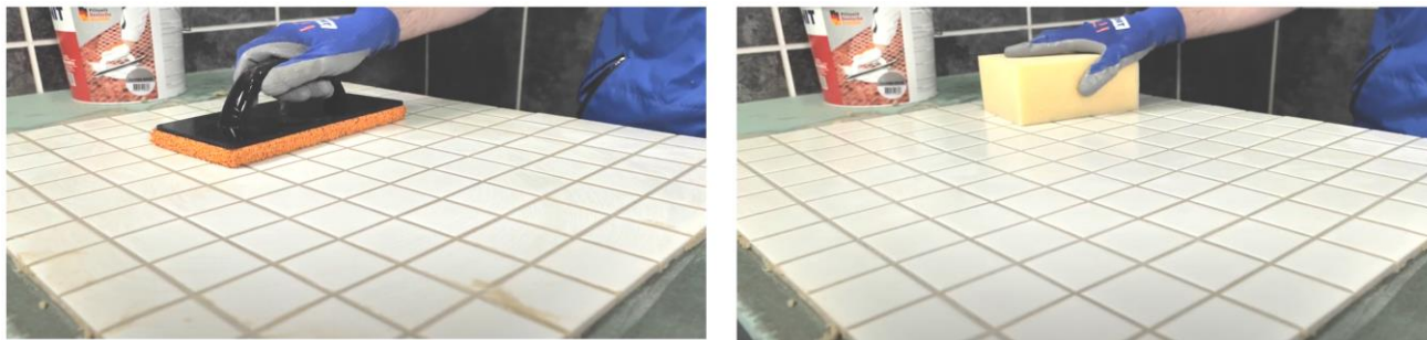
Рис. 27. Диагональными движениями шпателя убрать с поверхности плитки излишки затирки
