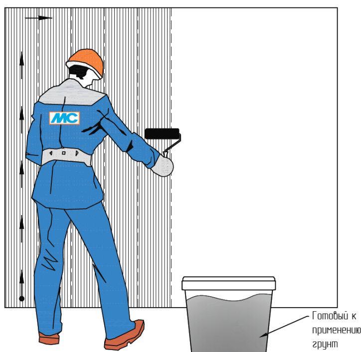
Рис. 29. Схема организации работ по нанесению грунта на основание
