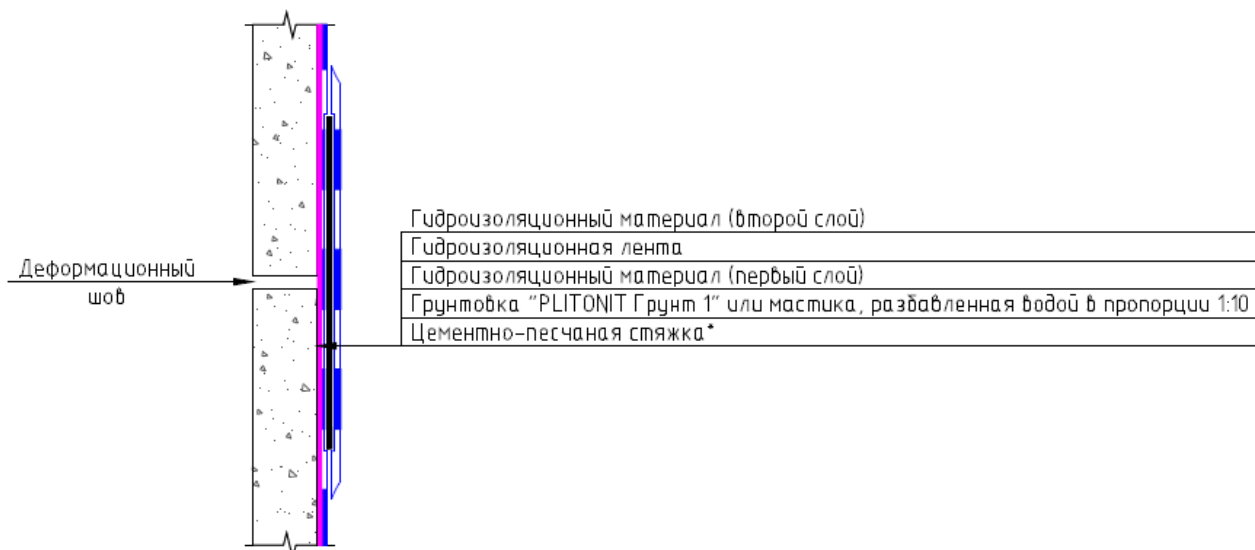
Рис.32.3. Конструктивный разрез №3.
