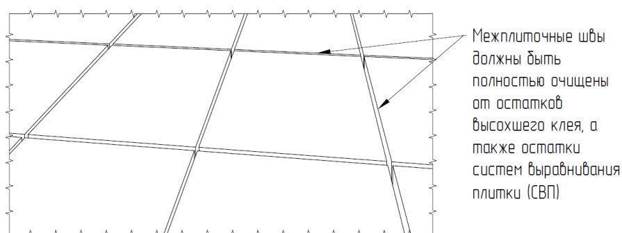
Рис. 36. Подготовка межплиточных швов
