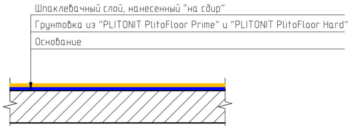
Рис.12. Конструктивный разрез №5.
