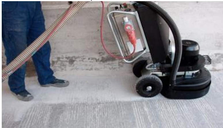
Рис.5. Очистка основания.
