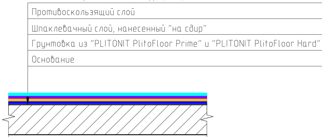
Рис.14. Конструктивный разрез №6.
