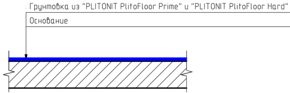
Рис.11. Конструктивный разрез №4.
