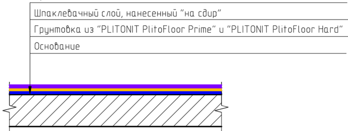
Рис.13. Конструктивный разрез №6.
