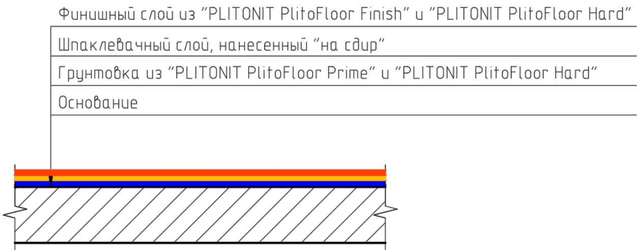
Рис.8. Конструктивный разрез №3.
