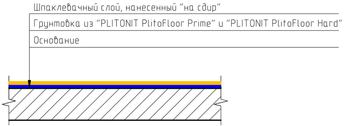
Рис.7. Конструктивный разрез №2.
