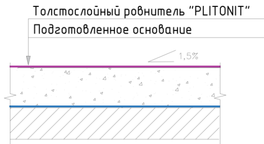
Сечение готового покрытия толстослойного ровнителя.
