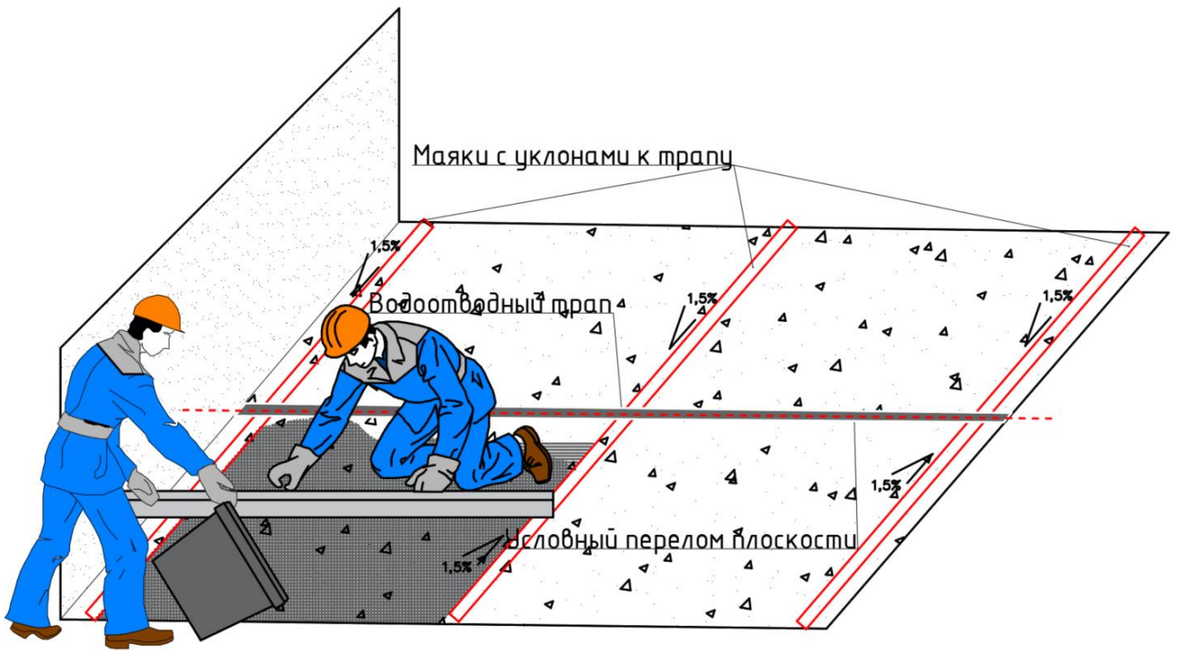
Вариант 2. Уклон к щелевидному трапу с одним переломом плоскости.
