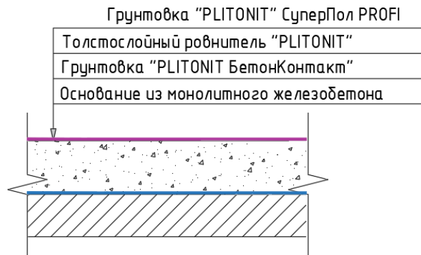
Сечение готового огрунтованного покрытия.
