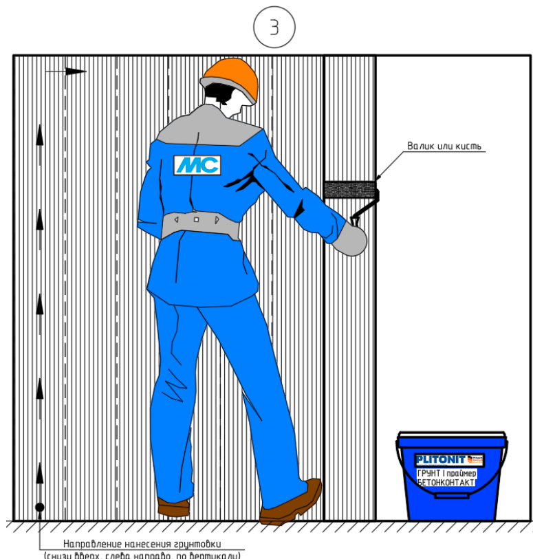
Рис. 17. Последовательность работ
