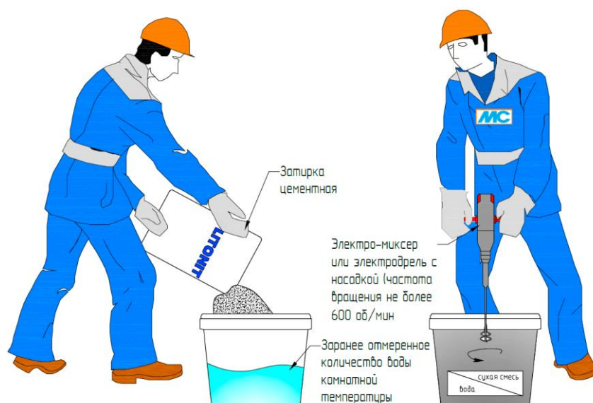
Рис. 33. Приготовление состава
