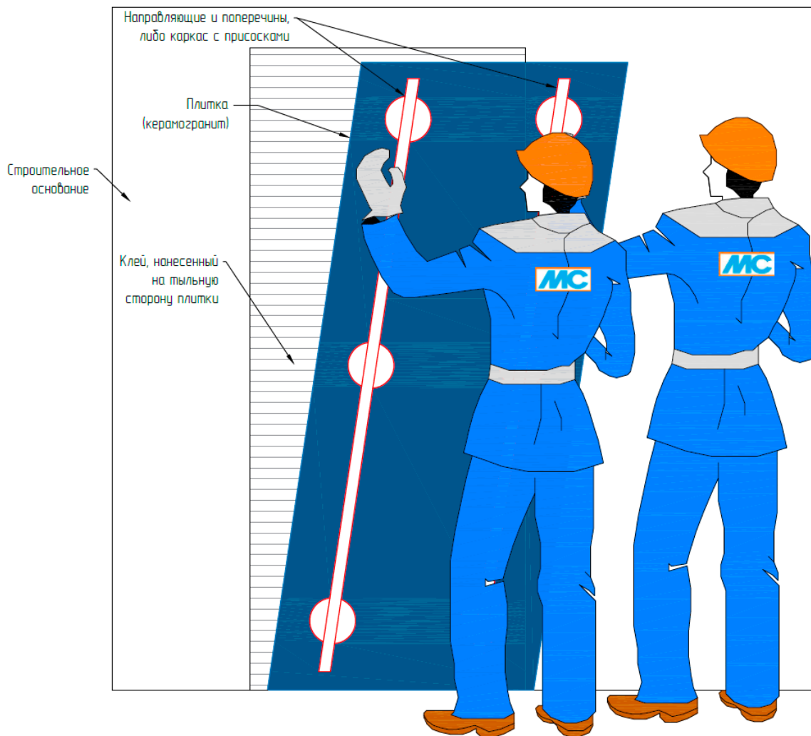
Рис. 25. Монтаж крупноформатного керамогранита
