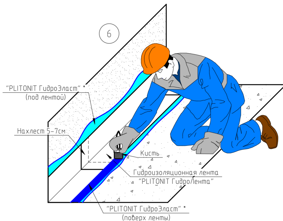
Рис.19. Последовательность работ, где: 1 - проверка ровности основания контрольной рейкой (аналогично для горизонтальной поверхности); 2 – размешивание емкости с мастикой; 3 – нанесение первого слоя мастики, разбавленной водой в пропорции 1:10, на основание; 4 – нанесение гидроизоляции на поверхность (аналогично для горизонтальной поверхности); 5 – укладка гидроизоляционной ленты на поверхность, предварительно обработанную «PLITONIT ГидроЭласт» или «PLITONIT WaterProof Standard»; 6 – поверхностная обработка ленты мастикой «PLITONIT ГидроЭласт» или «PLITONIT WaterProof Standard».
