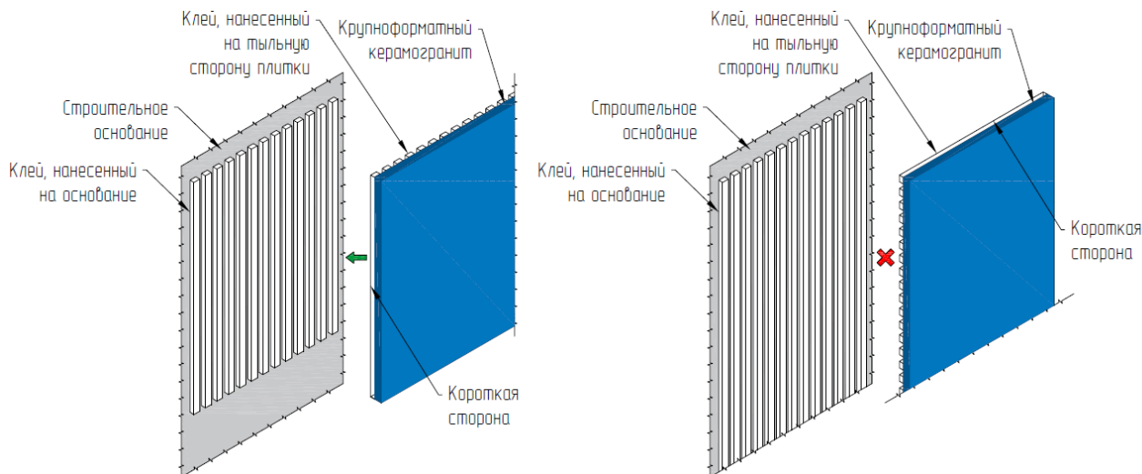
Рис. 21. Клей следует наносить в одном направлении на основание и на плитку
