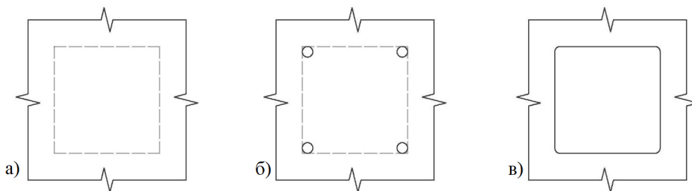
Рис. 24. Резка прямоугольных отверстий
