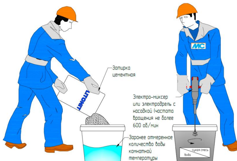
Рис. 29. Приготовление состава
