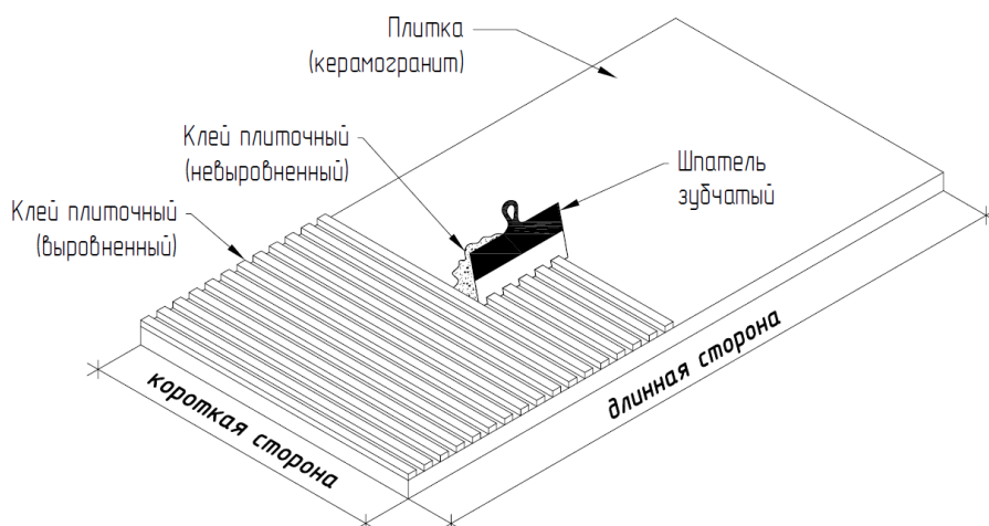
Рис. 20. Нанесение плиточного клея на плитку
