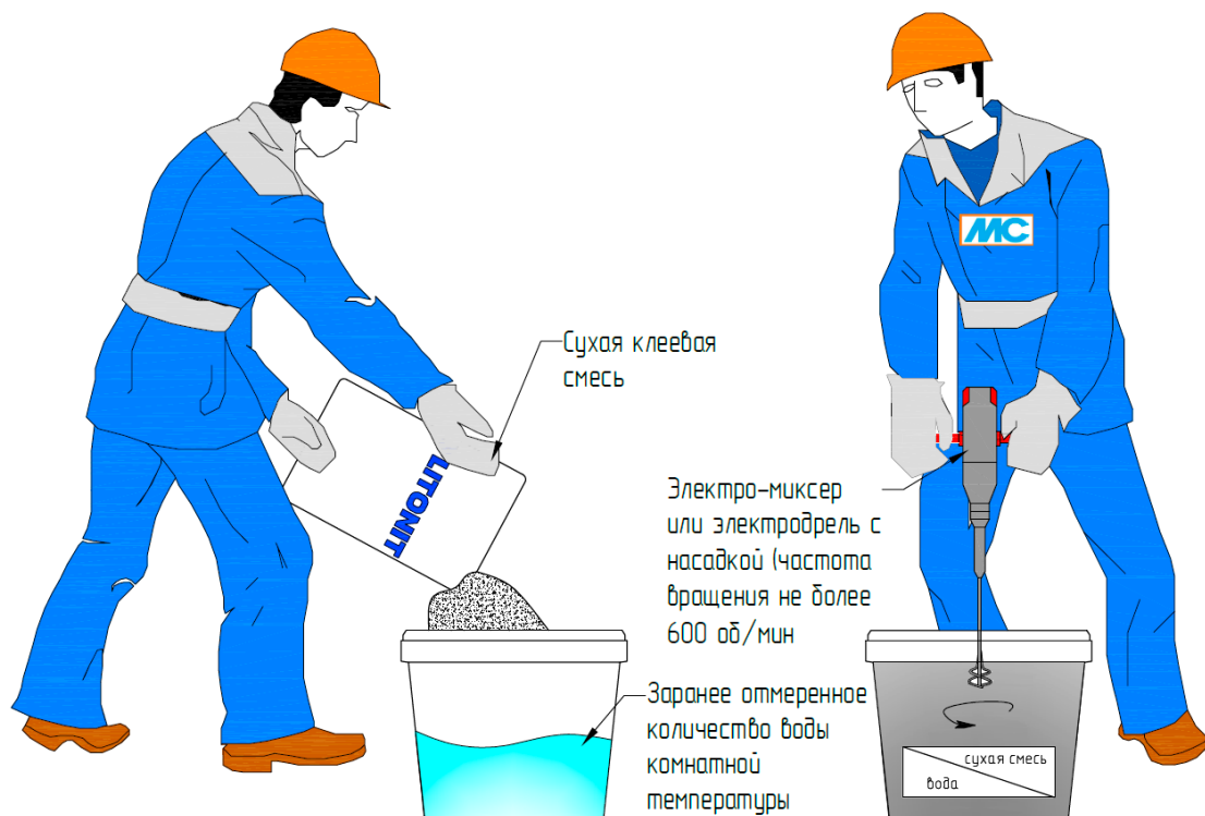
Рис. 10. Организация работ по затворению сухой клеевой смеси
