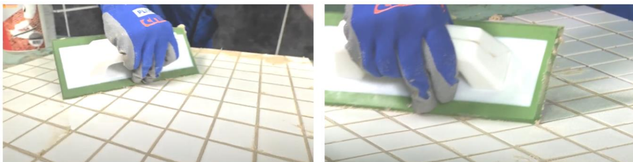
Рис. 15. Диагональными движениями шпателя убрать с поверхности плитки излишки затирки
