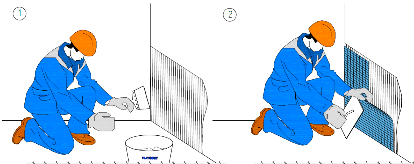
Рис. 11. Организация работ по приклеиванию мозаики
