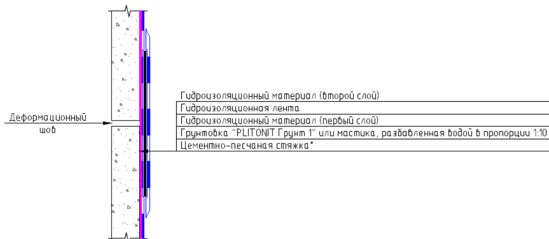
Рис.18.3. Конструктивный разрез №3.
