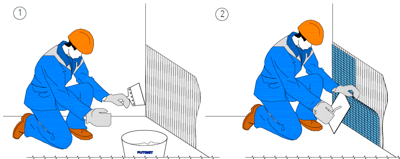
Рис. 15. Организация работ по приклеиванию мозаики
