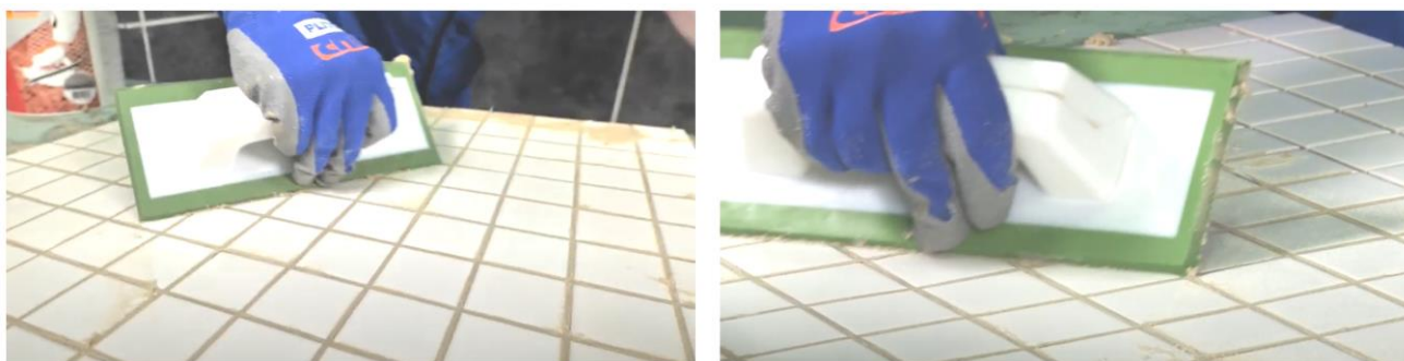
Рис. 19. Диагональными движениями шпателя убрать с поверхности плитки излишки затирки
