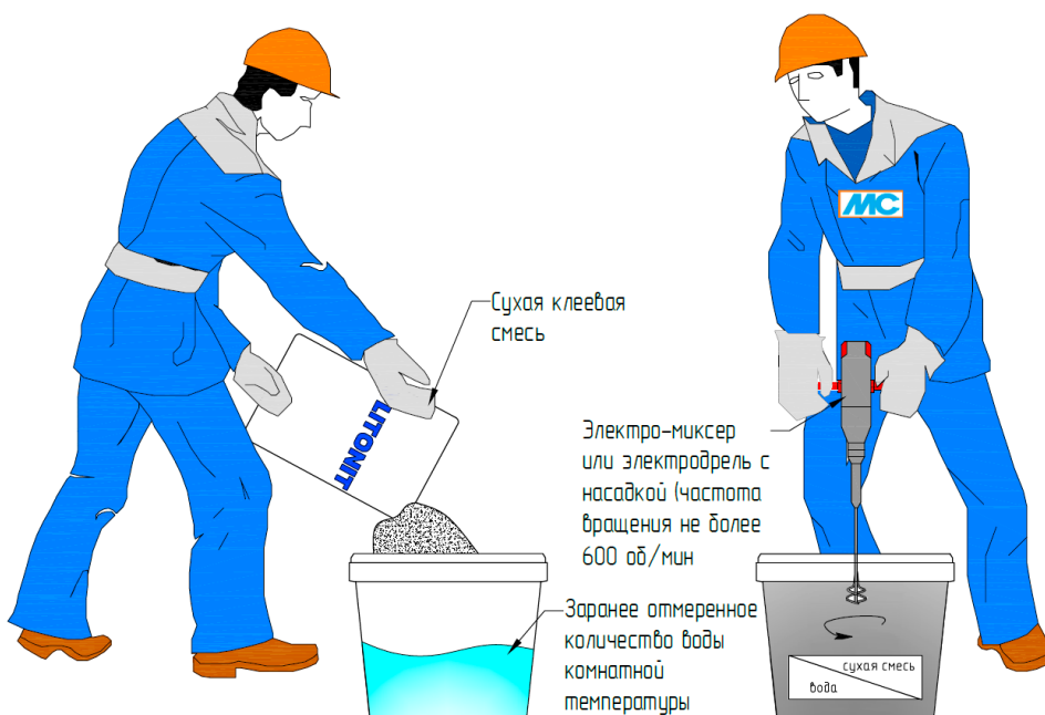
Рис. 14. Организация работ по затворению сухой клеевой смеси
