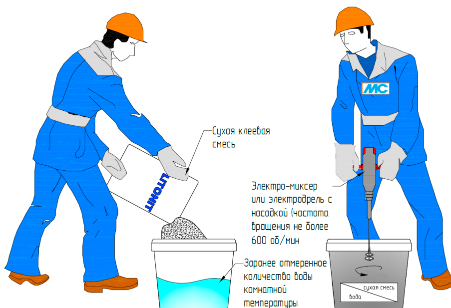
Рис. 27. Организация работ по затворению сухой клеевой смеси
