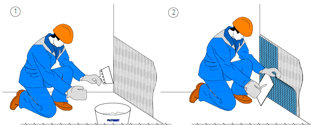
Рис. 22. Организация работ по приклеиванию мозаики
