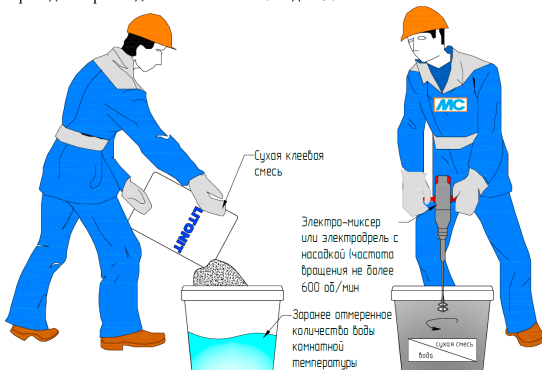
Рис. 21. Организация работ по затворению сухой клеевой смеси
