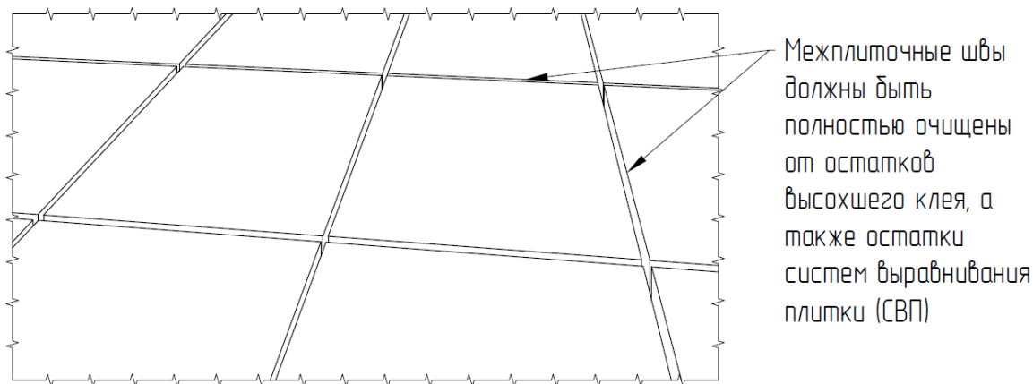
Рис. 23. Подготовка межплиточных швов
