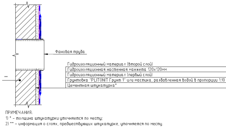
Рис.17.2. Конструктивный разрез №2.
