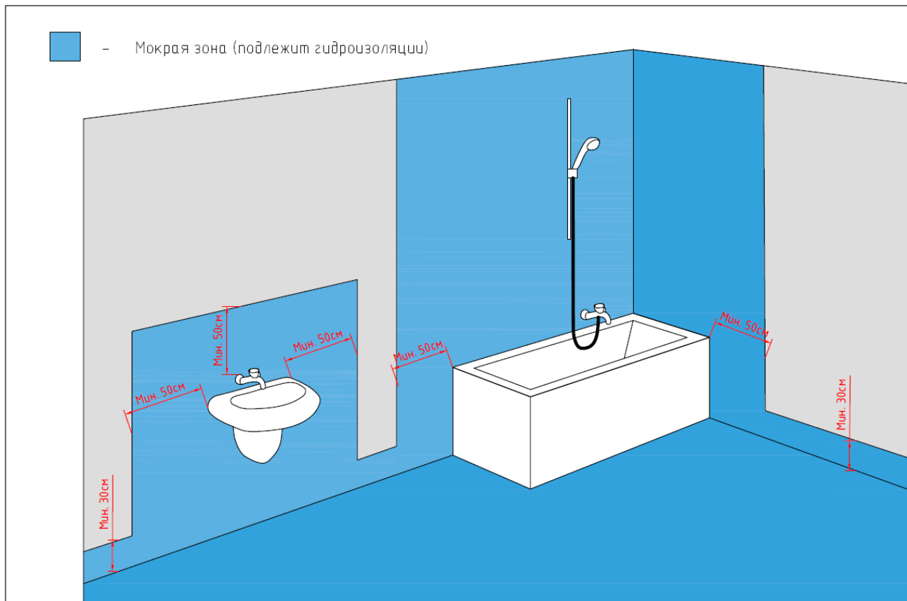
Рис. 18.2 Мокрые зоны внутри влажных помещений, подлежащие гидроизоляции.
