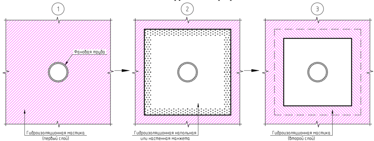
Рис.17.4. Последовательность нанесения гидроизоляционной манжеты.
