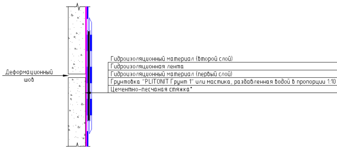
Рис.17.3. Конструктивный разрез №3.
