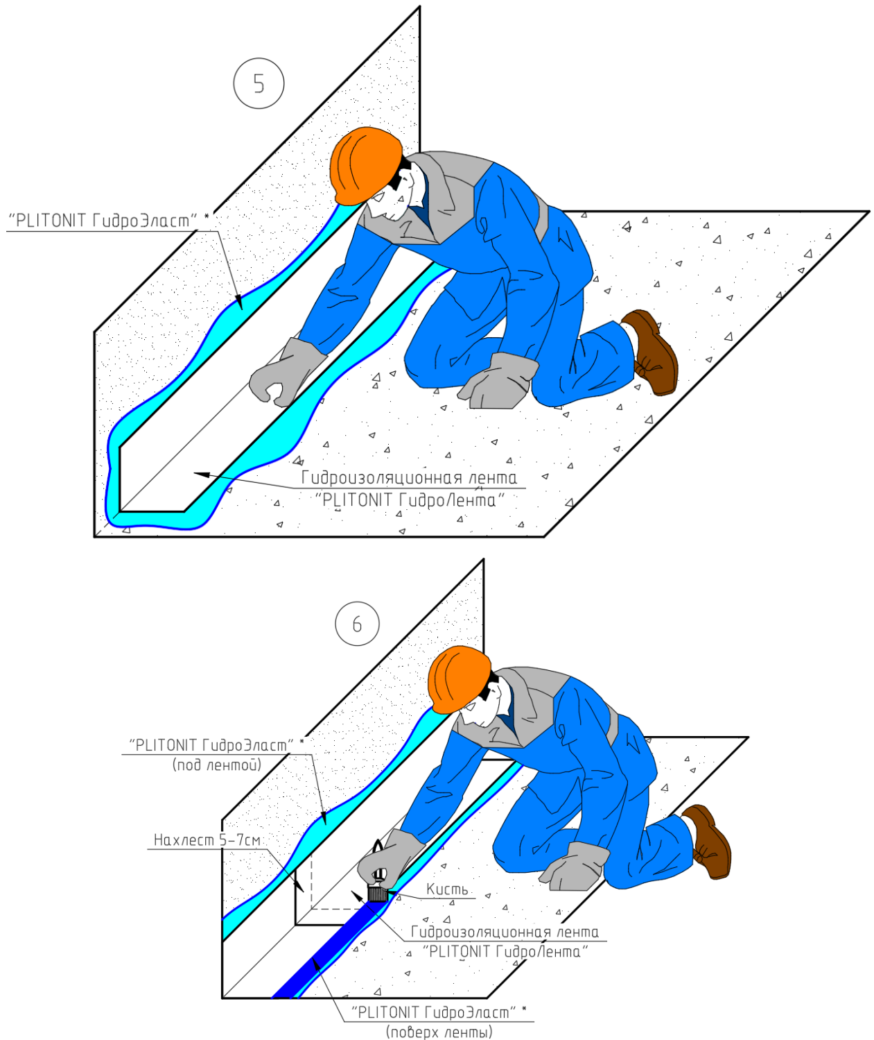
Рис.18.1. Последовательность работ (на стенах работа в аналогичном порядке), где: 1 - проверка ровности основания контрольной рейкой (аналогично для горизонтальной поверхности); 2 - размешивание емкости с мастикой; 3 - нанесение первого слоя мастики, разбавленной водой в пропорции 1:10, на основание; 4 - нанесение гидроизоляции на поверхность (аналогично для горизонтальной поверхности); 5 - укладка гидроизоляционной ленты на поверхность, предварительно обработанную «PLITONIT ГидроЭласт» или «PLITONIT WaterProof Standard»; 6 - поверхностная обработка ленты мастикой «PLITONIT ГидроЭласт» или «PLITONIT WaterProof Standard».
