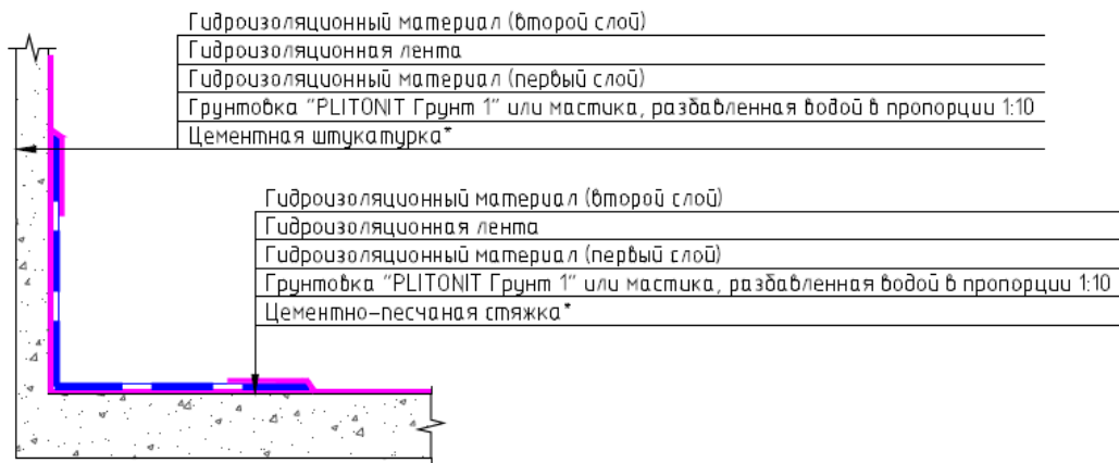
Разрез 1-1
