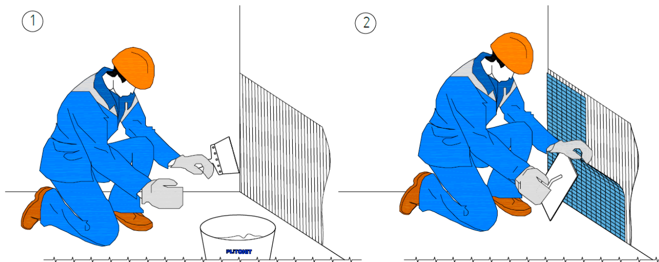
Рис. 6. Организация работ по приклеиванию мозаики
