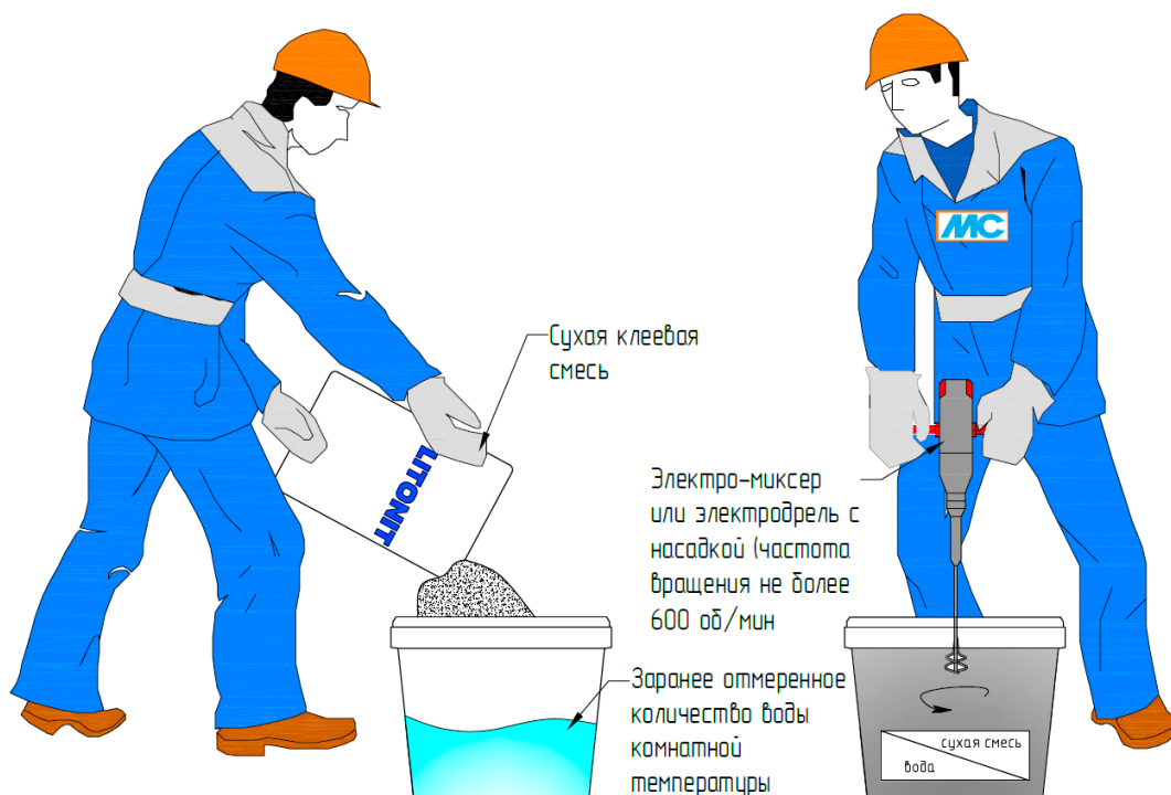
Рис. 3. Организация работ по затворению сухой клеевой смеси
