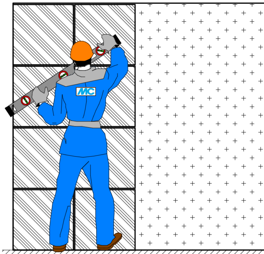
Рис.5. Последовательность работ, где: 1 – приготовление клеевой смеси; 2, 3 – нанесение клеевой смеси на основание (захватками); 4, 5 – приклеивание керамогранитной плитки на стену (захватками); 6 – проверка облицовки при помощи уровня.
