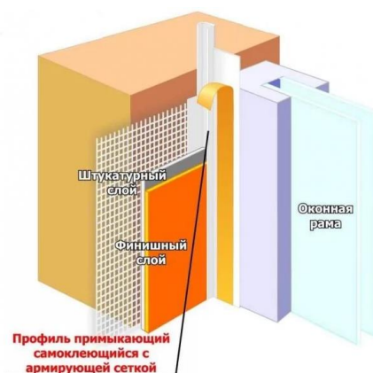
Рис.25. Профиль примыкающий с армирующей сеткой
