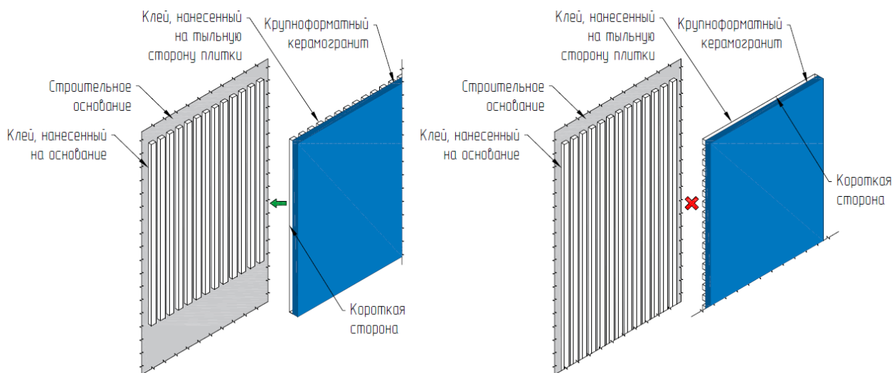
Рис. 35. Клей следует наносить в одном направлении на основание и на плитку
