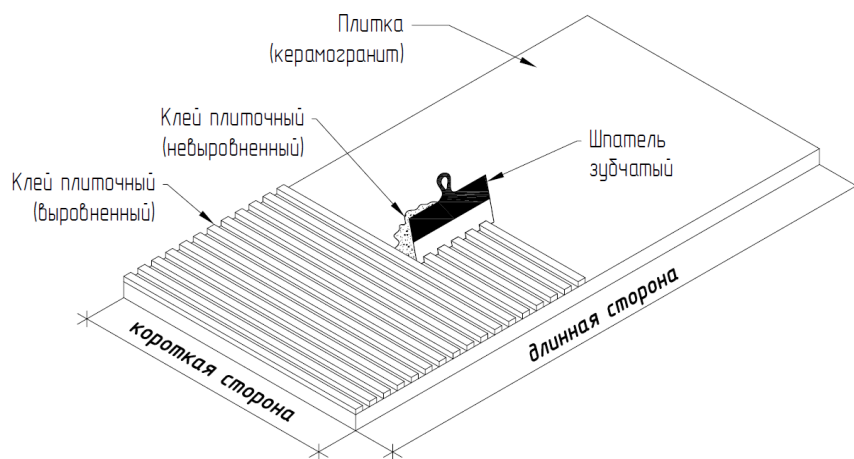
Рис. 34. Нанесение плиточного клея на плиту
