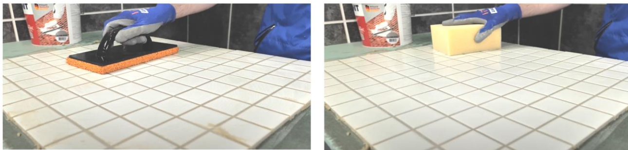
Рис. 44. Диагональными движениями шпателя убрать с поверхности плитки излишки затирки
