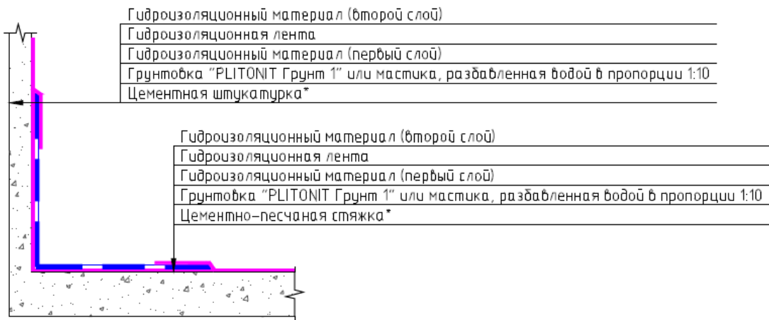
Разрез 1-1
