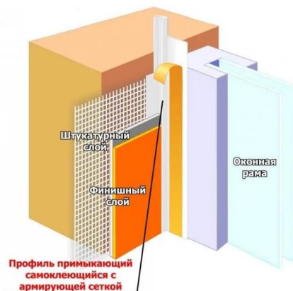
Рис.26. Профиль примыкающий с армирующей сеткой
