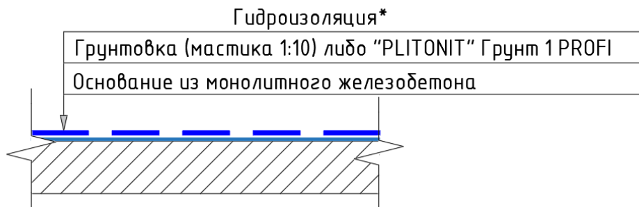
Сечение готового покрытия гидроизоляции.
