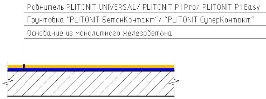
Рис.11. Конструктивный разрез №2.
