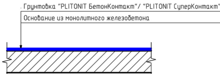
Рис.10. Конструктивный разрез №1.
