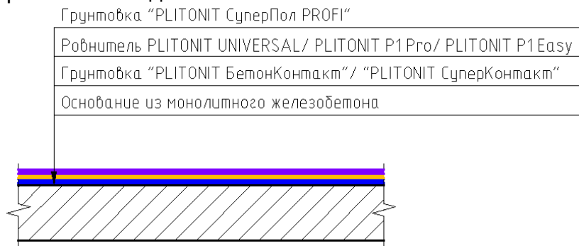
Рис.13. Конструктивный разрез №3.
