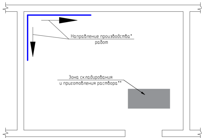
Рис.15. Схема организации работ (внутренние стены)
